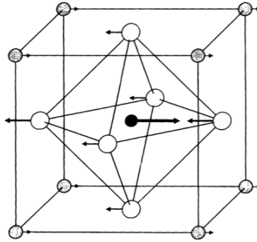
FIGURE 3 – Mode local polaire d'une pérovskite cubique. Les flèches donnent les déplacements relatifs qui composent la coordonnée collective \mathbf{u}_i [16].
