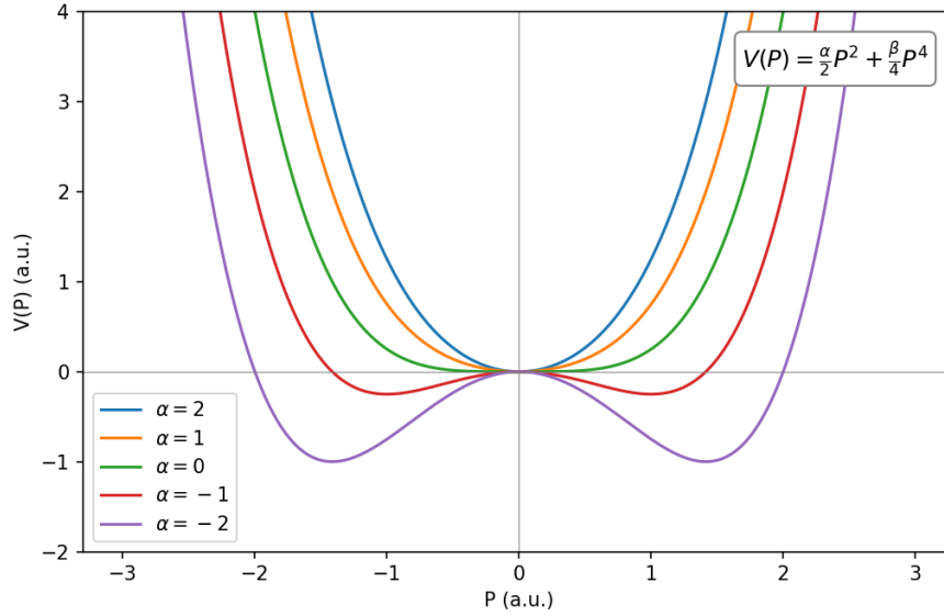
FIGURE 2 – Potentiel local de Landau V(P) = \alpha P^2/2 + \beta P^4/4 pour plusieurs valeurs de \alpha (ici \beta > 0 ). L'abscisse représente une composante du paramètre d'ordre local P(\mathbf{x}) à position fixée ; elle ne représente pas une dépendance spatiale. Le passage de \alpha > 0 à \alpha < 0 transforme le puits unique paraélectrique en deux minima ferroélectriques dégénérés. Schéma de l'auteur.
