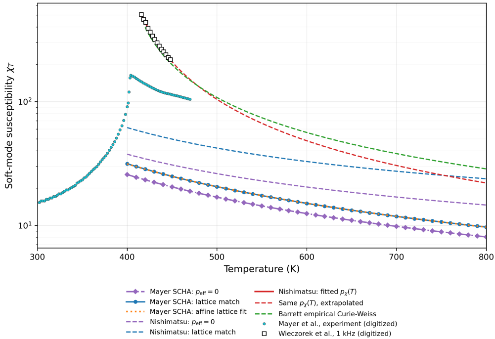
FIGURE 7 – Comparaison de la susceptibilité du mode mou pour les paramètres de Mayer. Les points sont des mesures numérisées ; les courbes continues ou pointillées sont des calculs ou des reconstructions empiriques. Les segments hors intervalle expérimental sont des extrapolations. Données et potentiel : Mayer et al. [22].
