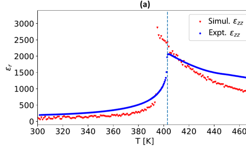
FIGURE 6 – Permittivit  calcul e par dynamique mol culaire classique avec le potentiel effectif enrichi de Mayer et al. Cette r f rence montre que l’enrichissement par les modes optiques secondaires rapproche fortement la tendance calcul e de la r ponse exp rimentale ; elle ne constitue pas une mesure directe. Adapt  de la figure 3(a) de la r f. [3].
