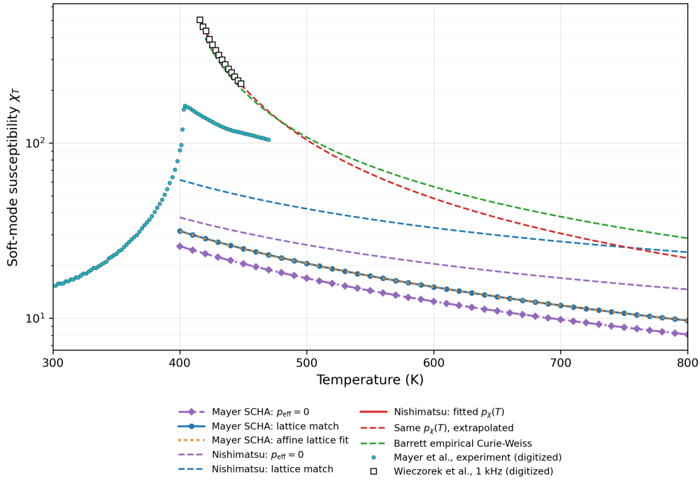
FIGURE 7 – Comparaison de la susceptibilit  du mode mou pour les param tres de Mayer. Les points sont des mesures num ris es ; les courbes continues ou pointill es sont des calculs ou des reconstructions empiriques. Les segments hors intervalle exp rimental sont des extrapolations. Donn es et potentiel : Mayer et al. [3].
