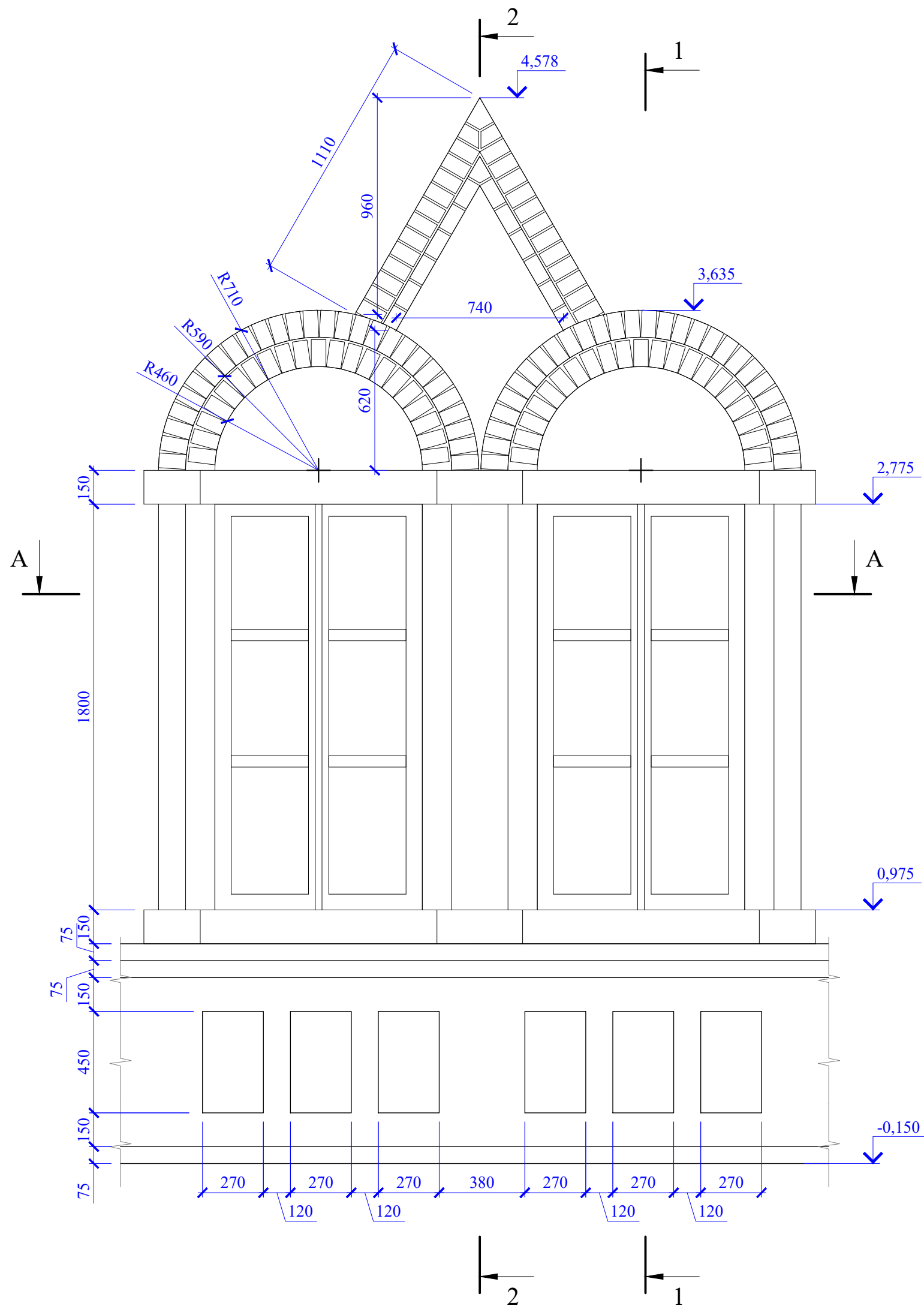
Фрагмент - наличники 1
