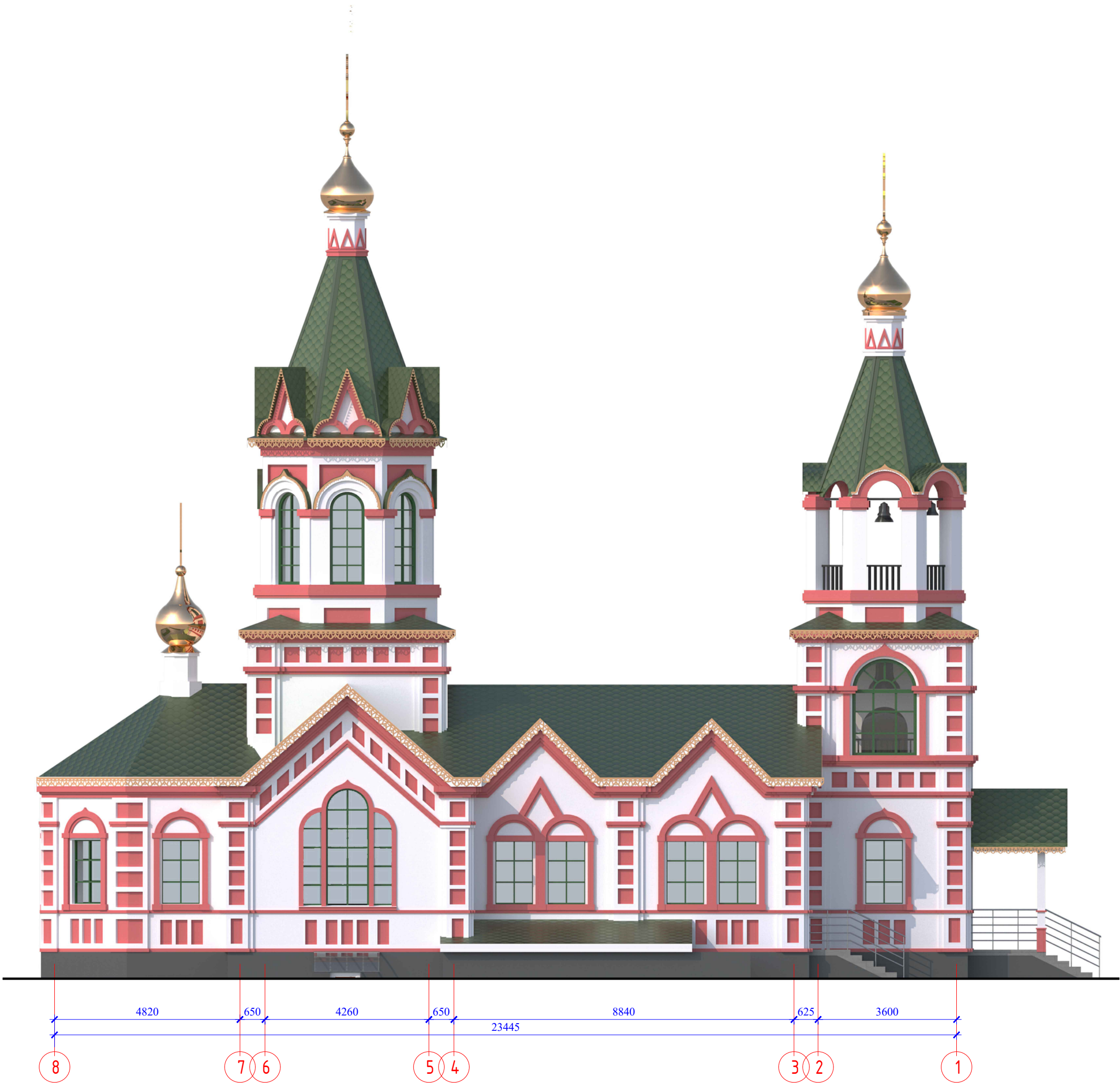
Фасад 8-1. М 1:100.
