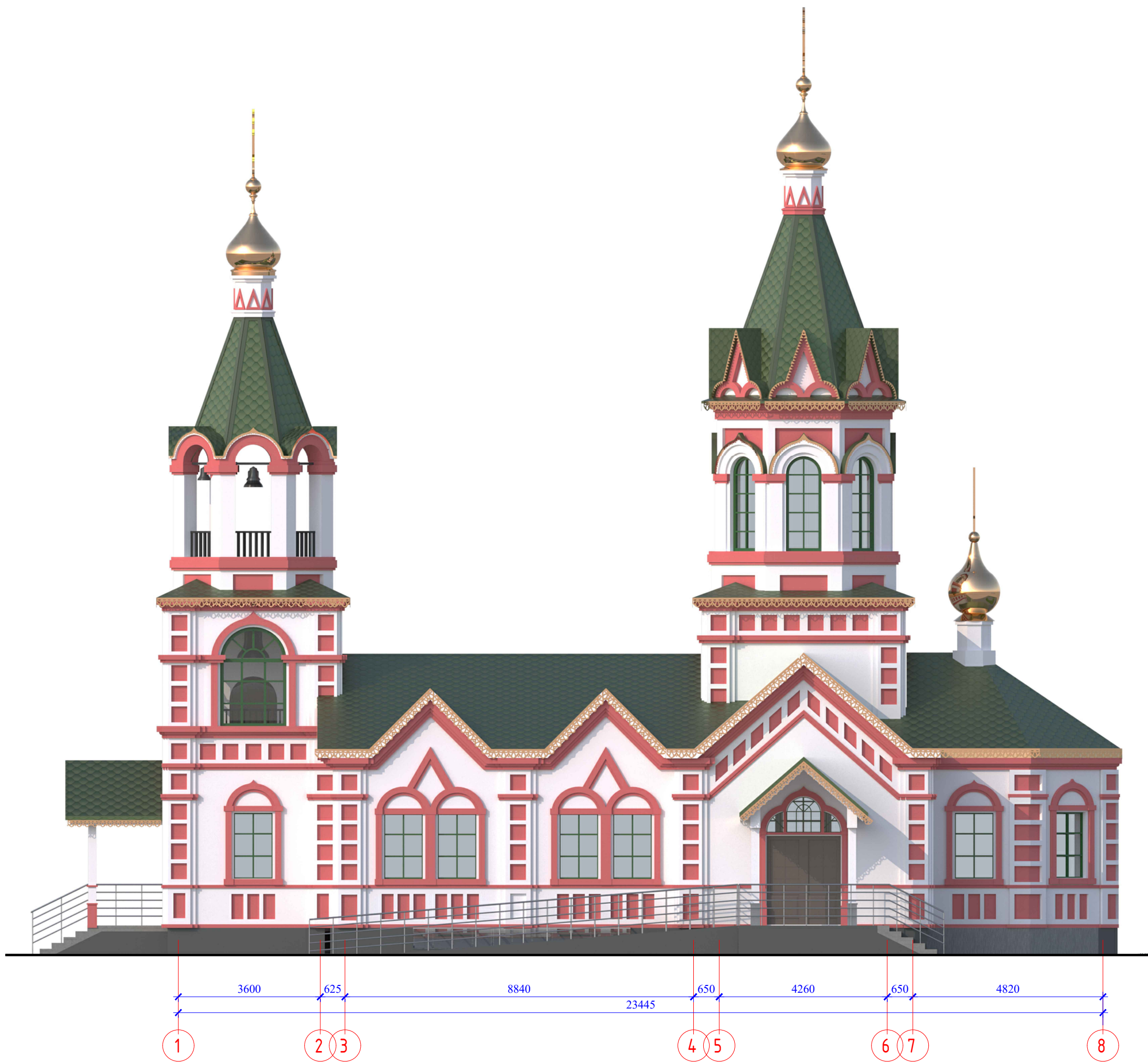
Фасад 1-8. М 1:100.
