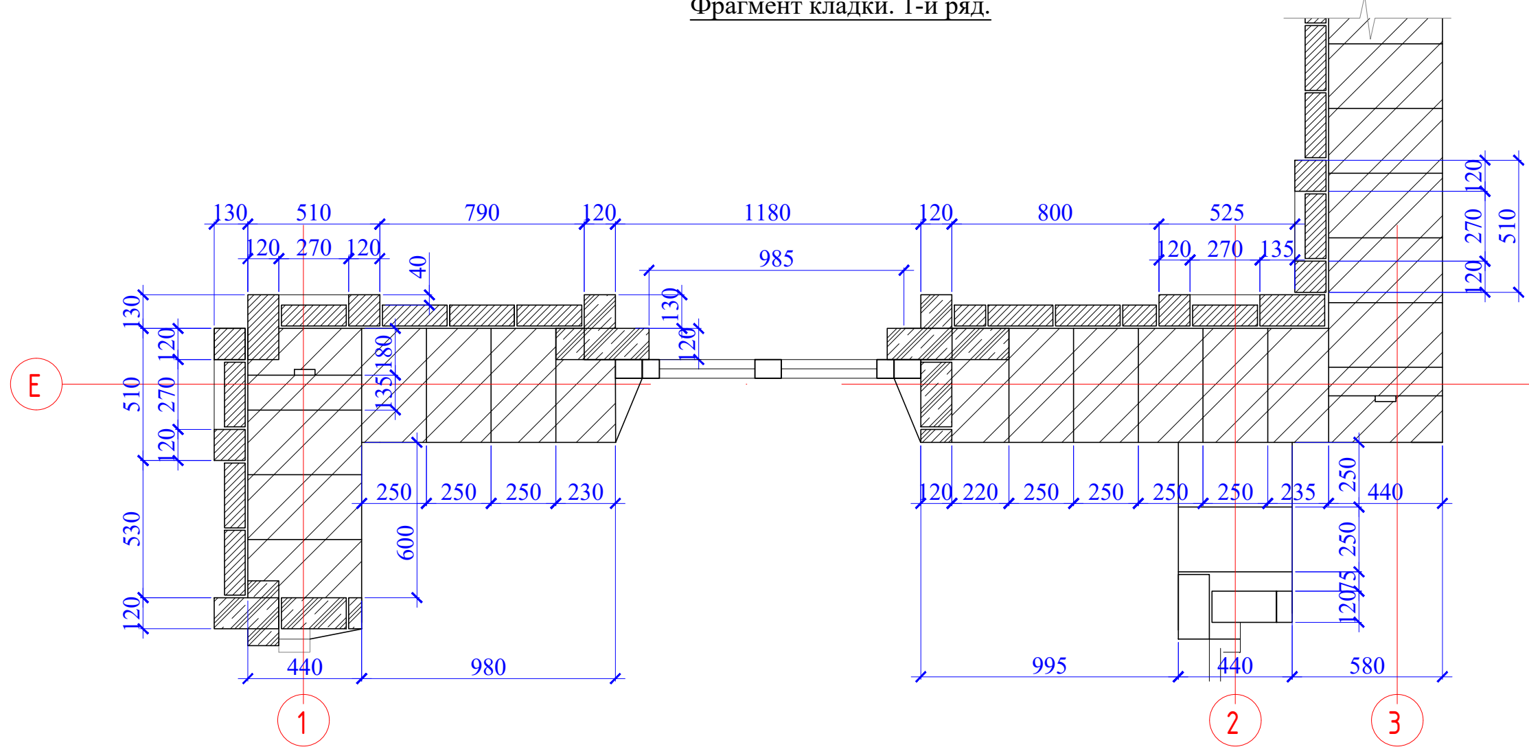
Фрагмент кладки. 1-й ряд.
