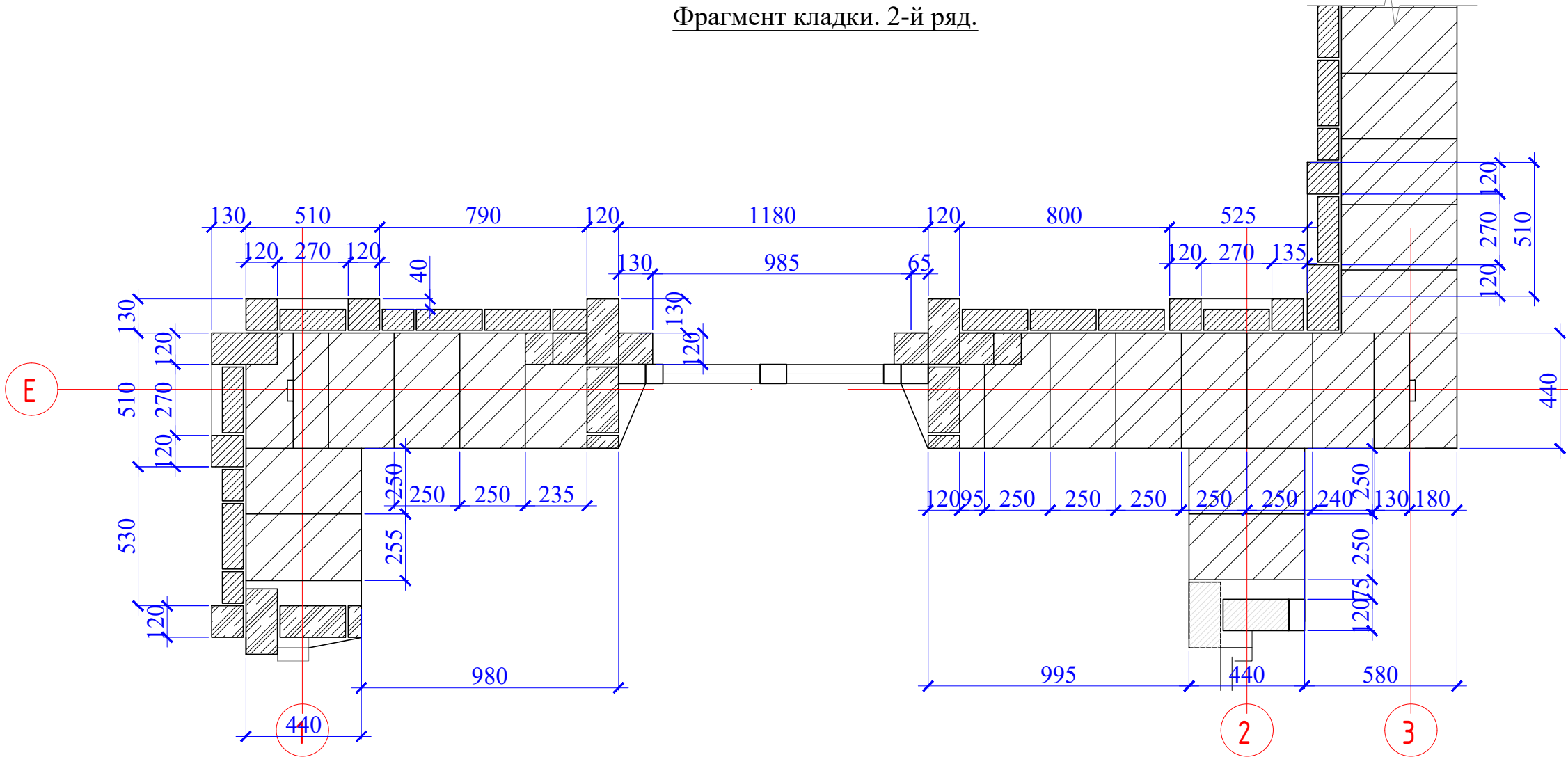
Фрагмент кладки. 2-й ряд.
