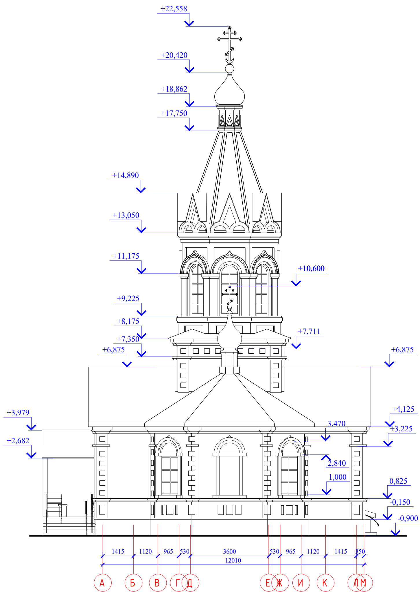
Фасад А-М. М 1:100.
