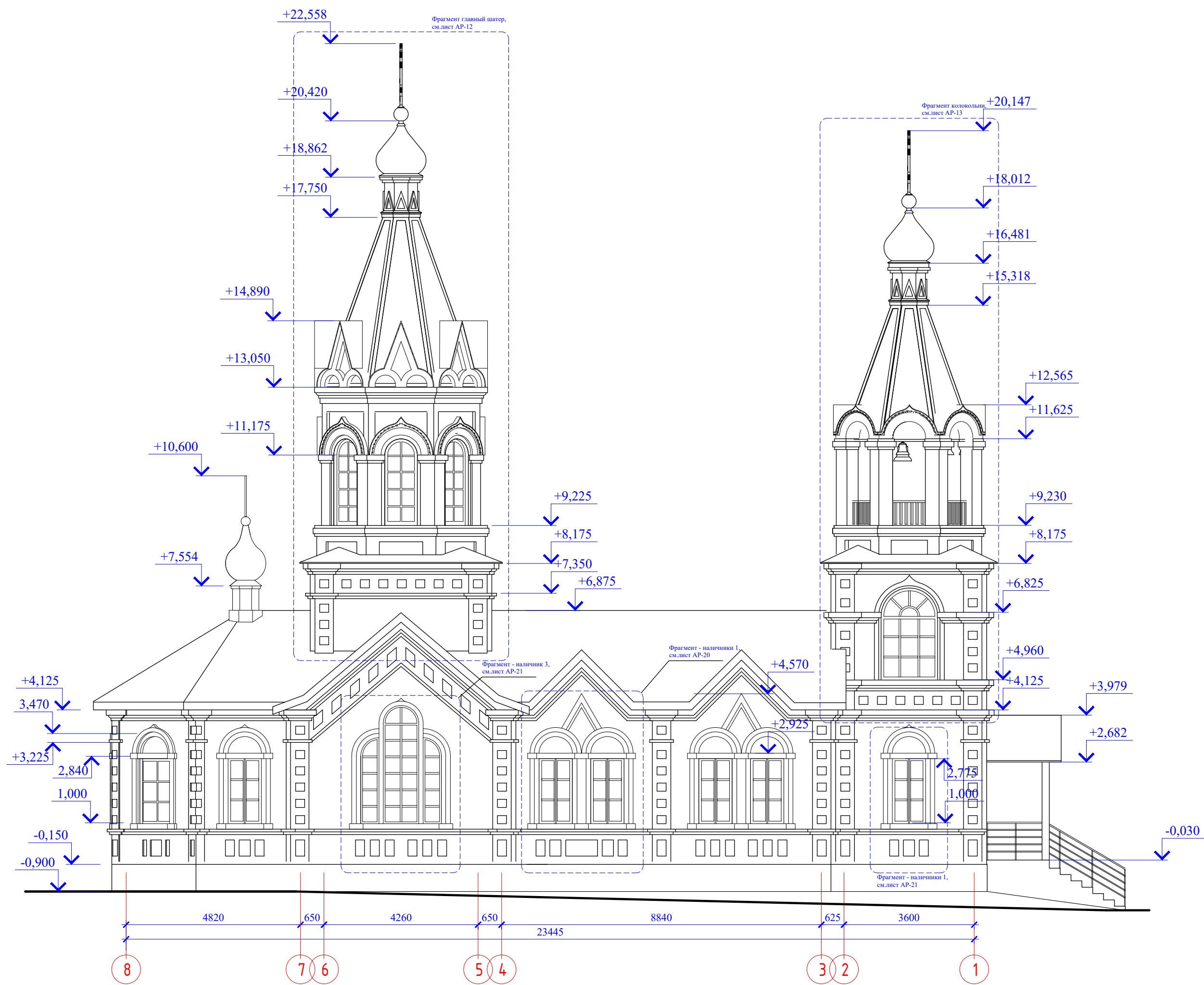
Фасад 8-1. М 1:100.
