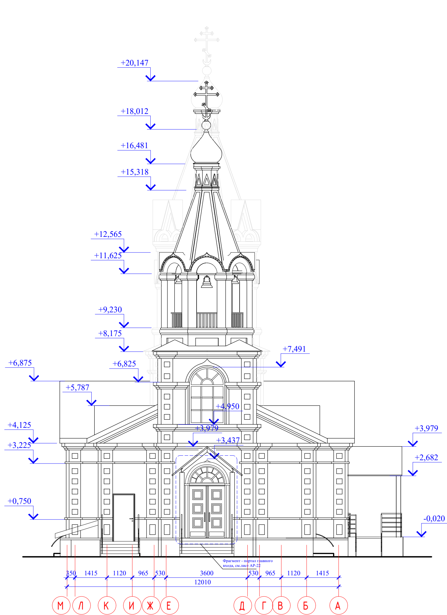
Фасад М-А. М 1:100.
