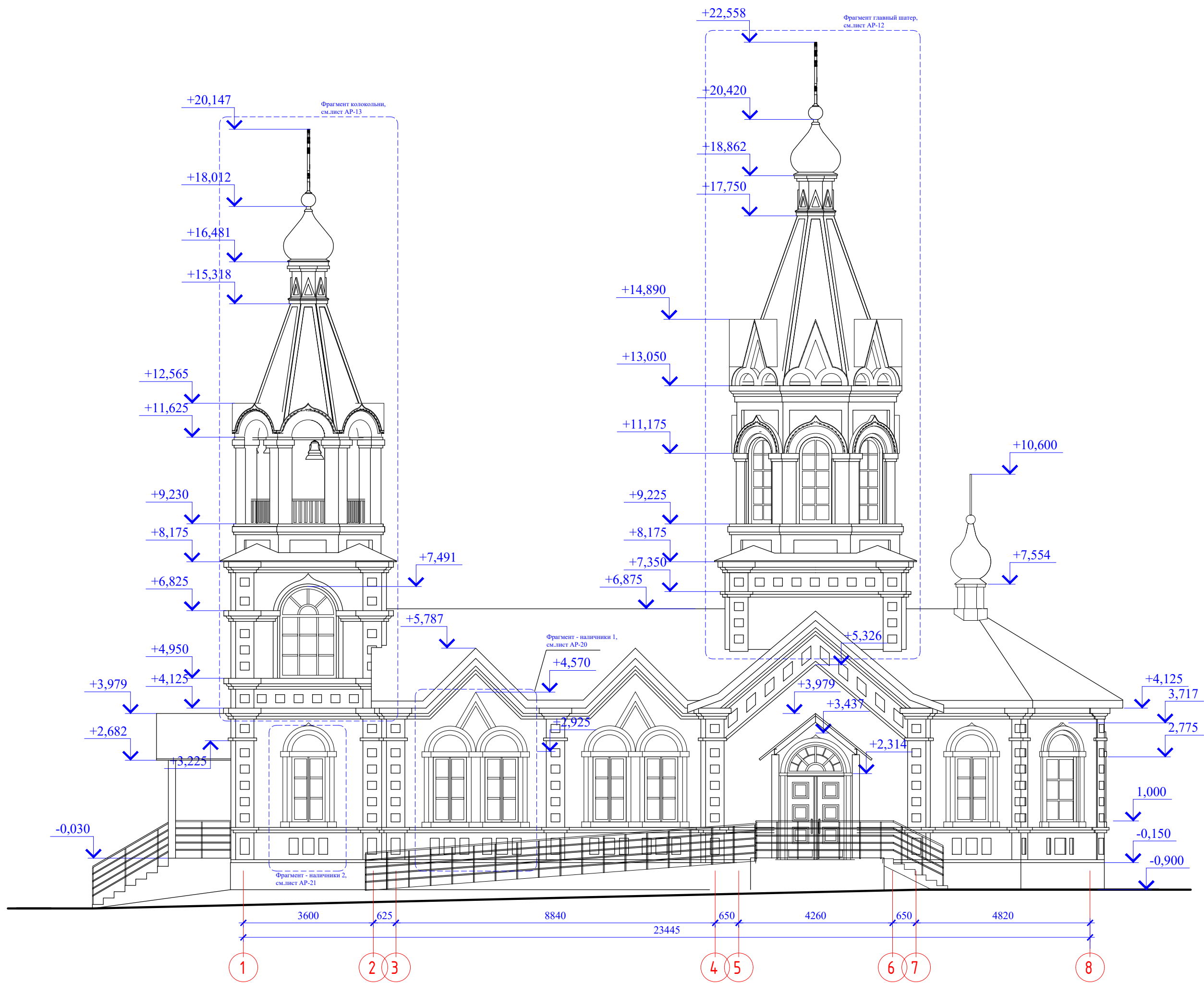
Фасад 1-8. М 1:100.
