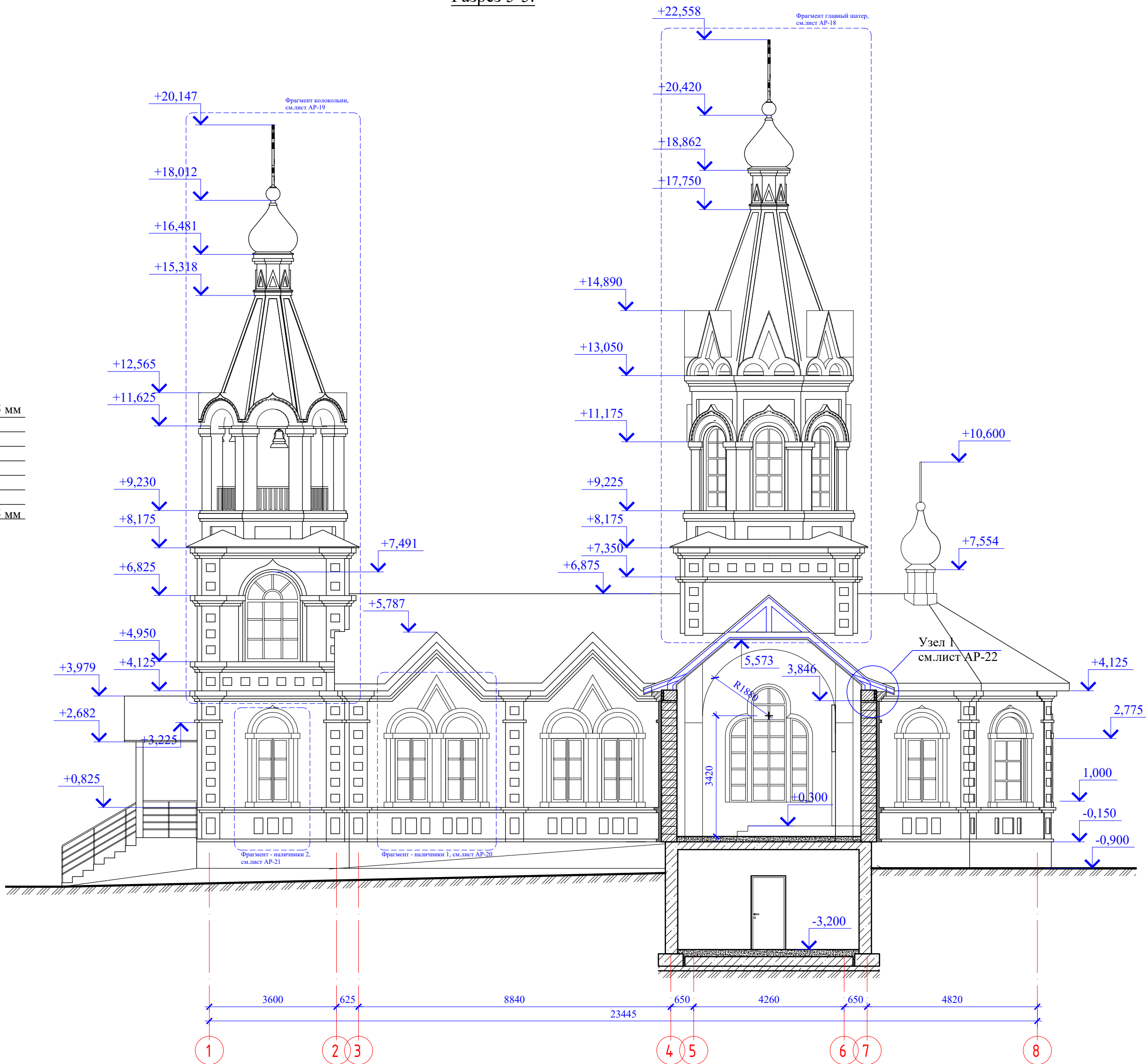
Разрез 5-5.
