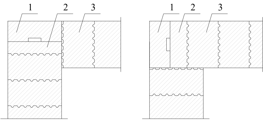
Схема кладки Parotherm 44
