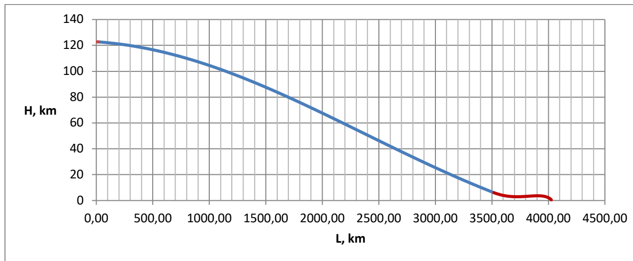
Рисунок 1 – Профиль траектории снижения. Красным цветом показаны активные участки
