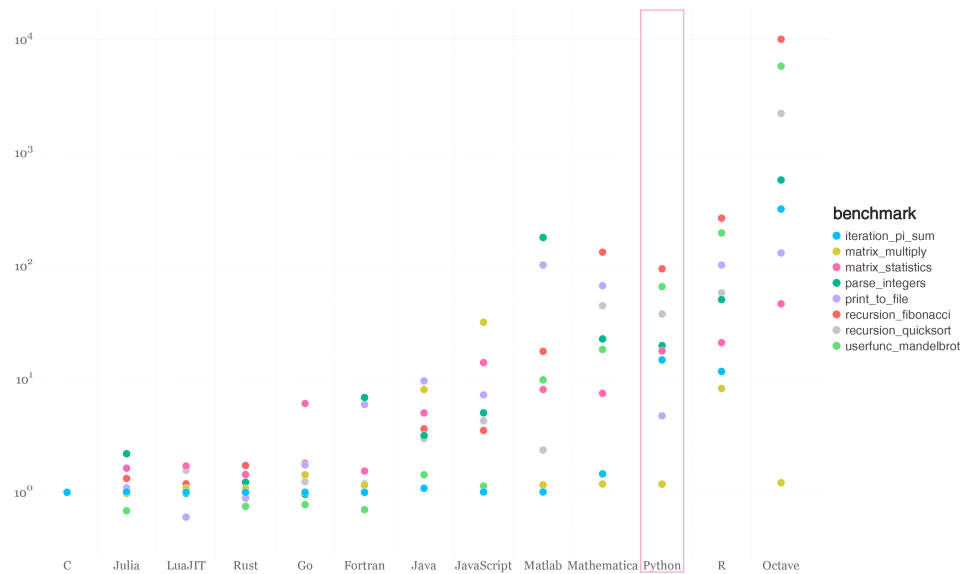
FIGURE 1.14 – Comparaison des temps de calcul entre le Python et d’autres langages de programmation avec différents algorithmes classiques
