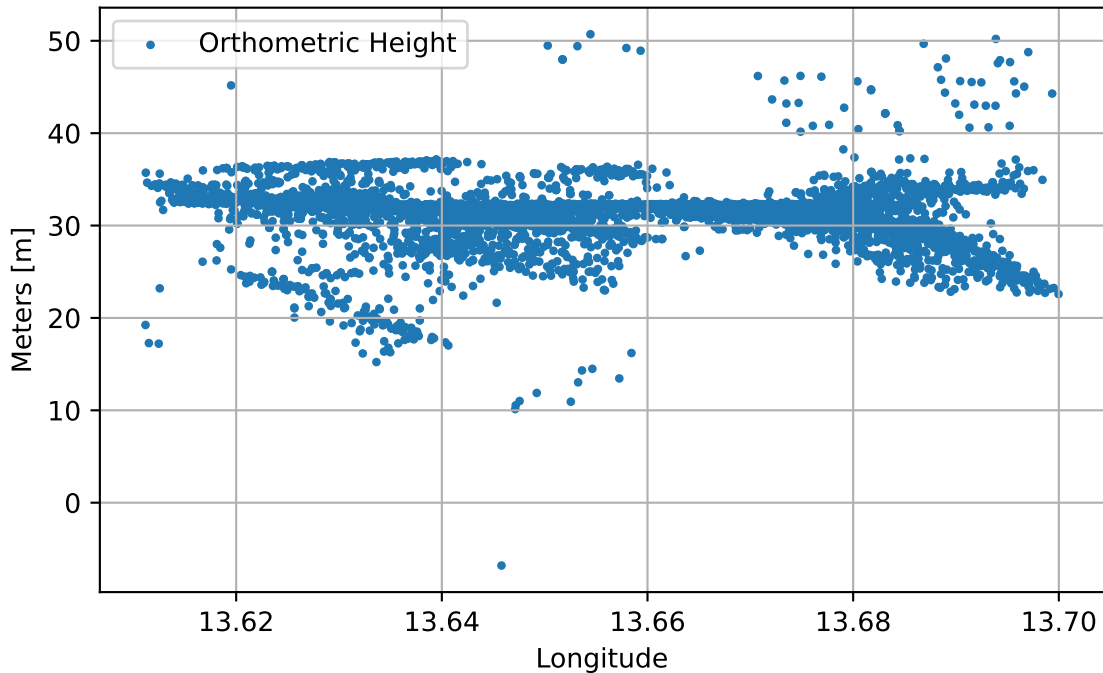
Orthometric Height over Longitude
