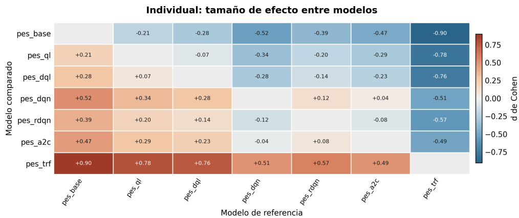
Figura C.2: Modelos individuales: d de Cohen entre pares de modelos en los 21 escenarios de generalización.
