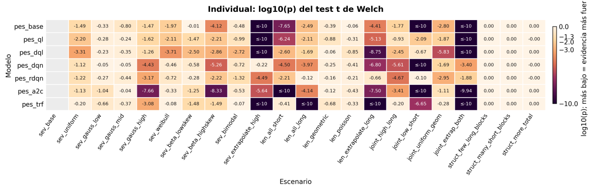
Figura C.1: Modelos individuales: \log_{10} p de Welch de cada escenario frente a la referencia del mismo modelo; los valores menores que -10 se muestran como \leq -10 .
