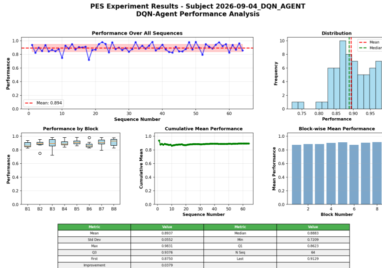
Figura 5.6: Resultados por secuencia de DQN (pes_dqn) en la referencia.
