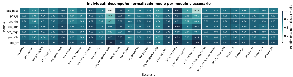
Figura 5.1: Modelos individuales: desempeño medio \bar{r} por modelo y escenario. La primera columna es la referencia. Las cinco columnas a la derecha de la línea vertical son las réplicas fuera de muestra.
