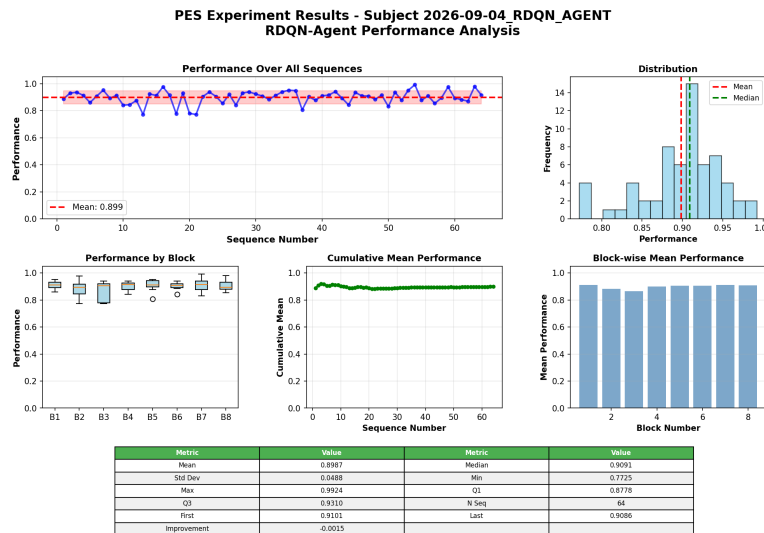
Figura 5.7: Resultados por secuencia del DQN recurrente (pes_rdqn) en la referencia.
