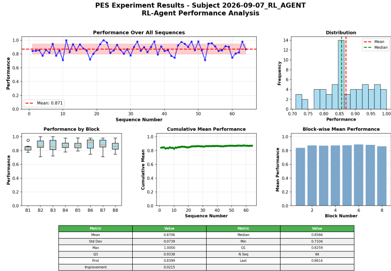
Figura 5.3: Resultados por secuencia de Q-Learning base (pes_base) en la referencia.
