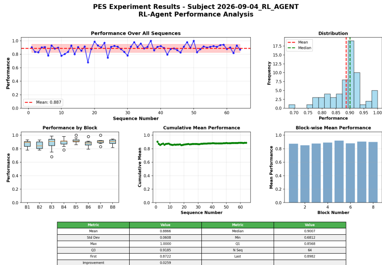
Figura 5.4: Resultados por secuencia de Q-Learning (pes_q1) en la referencia.
