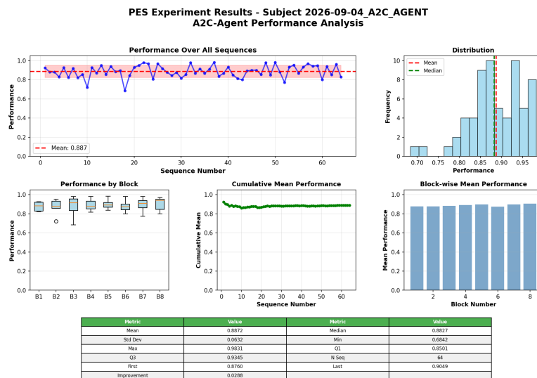
Figura 5.8: Resultados por secuencia de A2C (pes_a2c) en la referencia.
