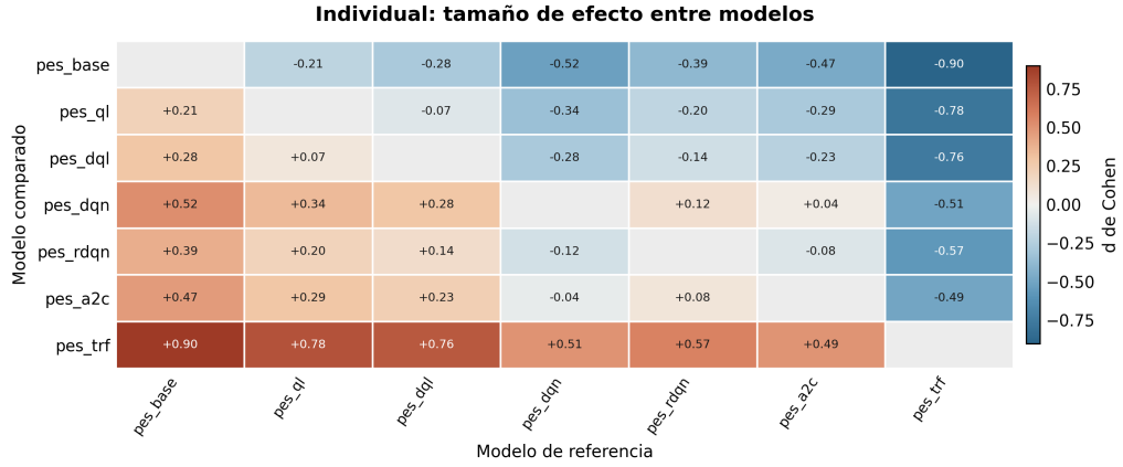
Figura C.2: Modelos individuales: d de Cohen entre pares de modelos en los 21 escenarios de generalización.
