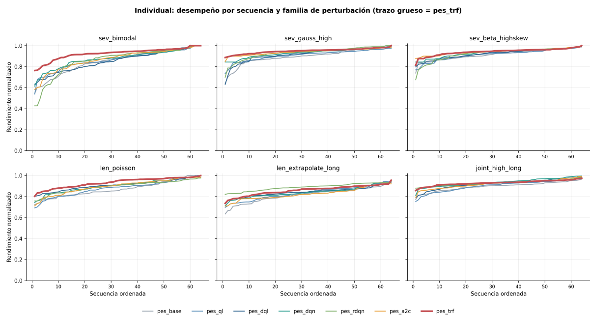
Figura 5.2: Desempeño por secuencia, ordenado de menor a mayor, en seis escenarios de generalización. Fila superior: severidad; fila inferior: longitud y conjunta. El trazo grueso corresponde al Transformer.
