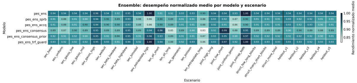
Figura 5.10: Ensamblas: desempeño medio \bar{r} por ensamble y escenario. La primera columna es la referencia. Las cinco columnas a la derecha de la línea vertical son las réplicas fuera de muestra.
