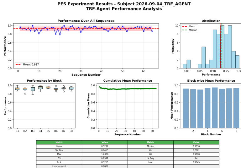
Figura 5.9: Resultados por secuencia del Transformer ( pes_trf ) en la referencia.
