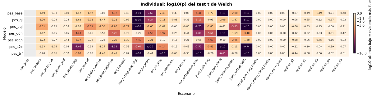
Figura C.1: Modelos individuales: \log_{10} p de Welch de cada escenario frente a la referencia del mismo modelo; los valores menores que -10 se muestran como \leq -10 . Las cinco columnas a la derecha de la línea vertical son las réplicas fuera de muestra.
