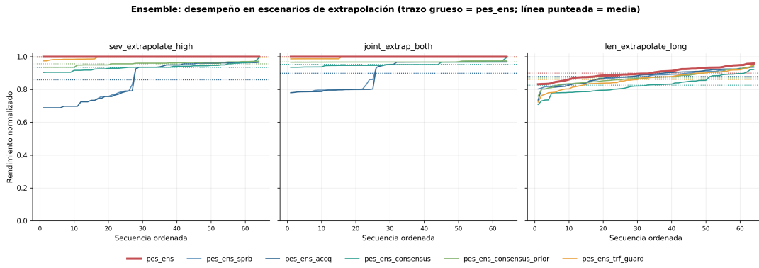
Figura 5.11: Desempeño por secuencia, ordenado de menor a mayor, de los seis ensambles en los escenarios fuera de rango; trazo grueso: ensemble ponderado; líneas punteadas: media de cada ensemble.
