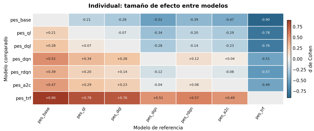
Figura 5.5: d de Cohen (Ecuación (2.18)) entre pares de modelos de la suite individual, calculada sobre los 21 escenarios de perturbación. Un valor positivo indica que el modelo de la fila supera en media al de la columna.
