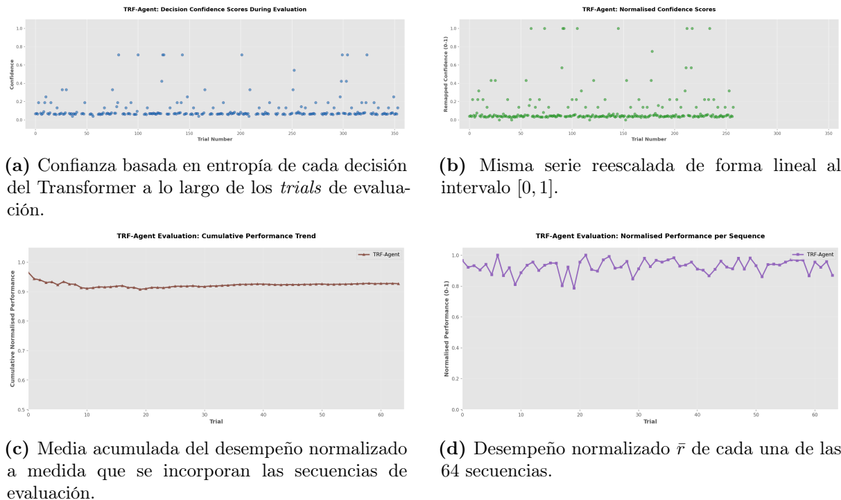
Figura 4.2: Variables registradas al evaluar el agente pes_trf tras su entrenamiento. Los paneles superiores muestran la confianza basada en entropía por decisión (cruda y reescalada a [0, 1] ); los paneles inferiores, la media acumulada y el desempeño normalizado por secuencia.
