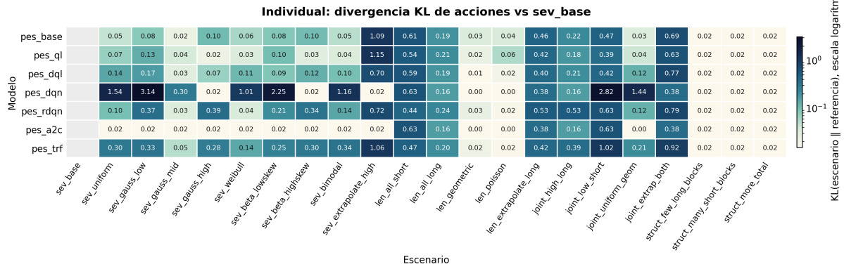
Figura 5.4: Suite individual: divergencia D_{KL} (Ecuación (2.20)) entre la distribución empírica de acciones de cada escenario y la de la referencia del mismo modelo. Mide el desplazamiento de la política, no el rendimiento.
