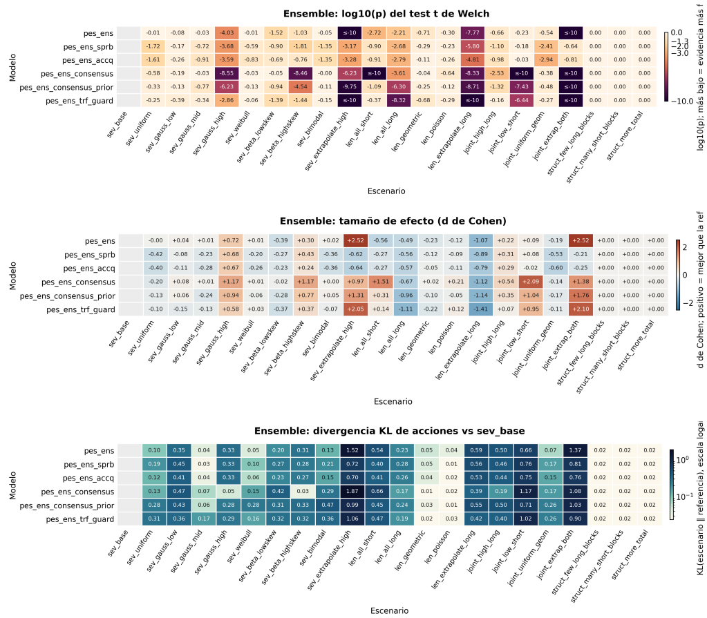
Figura C.4: Ensamble: \log_{10} p de Welch (arriba), d de Cohen (centro) y divergencia KL de acciones (abajo) de cada escenario frente a la referencia del mismo ensamble.
