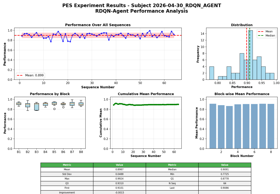
Figura 5.10: Desempeño por secuencia, distribución, estadísticos por bloque y resumen descriptivo de pes_rdn.
