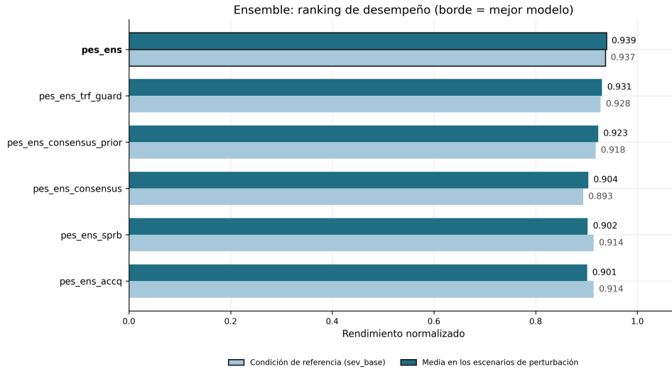
Figura 5.16: Media del desempeño normalizado en la condición de referencia y en los 21 escenarios de perturbación para las seis variantes de ensamble; el borde destaca a pes_ens .
