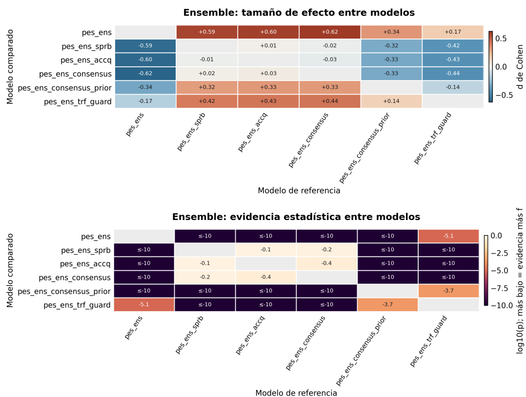
Figura 5.21: Contrastes pareados entre las seis variantes de ensemble: d de Cohen arriba y \log_{10} p de Welch abajo, calculados sobre los 21 escenarios de perturbación comunes y sus 64 secuencias.
