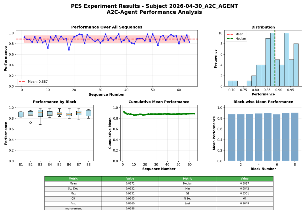
Figura 5.10: Desempeño por secuencia, distribución, estadísticos por bloque y resumen descriptivo de pes_a2c.
