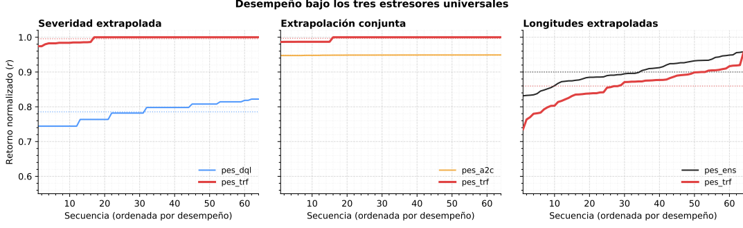
Figura 5.14: Curvas de desempeño por secuencia bajo los tres estresores universales, con las secuencias ordenadas de menor a mayor desempeño normalizado \bar{r} (Ec. (5.1)). Izquierda: severidad extrapolada ( pes_dql en azul, pes_trf en rojo). Centro: extrapolación conjunta ( pes_a2c en naranja, pes_trf en rojo; ambas trazas prácticamente planas indican una política sin sensibilidad al estresor). Derecha: longitudes extrapoladas ( pes_ens en negro, pes_trf en rojo). Las líneas punteadas marcan la media de cada modelo a lo largo de las 64 secuencias.
