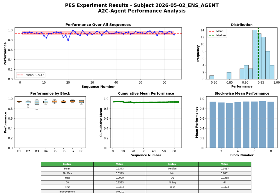
Figura 5.12: Desempeño por secuencia, distribución, estadísticos por bloque y resumen descriptivo de pes_ens.
