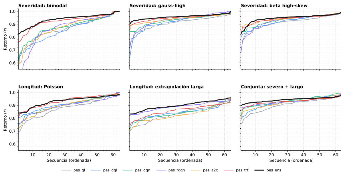
Figura 5.13: Curvas adicionales de desempeño por secuencia, organizadas por familia de perturbación. Fila superior: severidad ( sev_bimodal , sev_gauss_high , sev_beta_highskew ). Fila inferior: longitud ( len_poisson , len_extrapolate_long ) y combinación conjunta ( joint_high_long ). Cada panel ordena las n = 64 secuencias de menor a mayor desempeño normalizada \bar{r} (Ec. (5.1)) para los siete modelos evaluados. El modelo de referencia pes_base se excluye del conjunto optimizado al carecer de sintonización de hiperparámetros; el ensemble pes_ens se traza en negro y con trazo más grueso.
