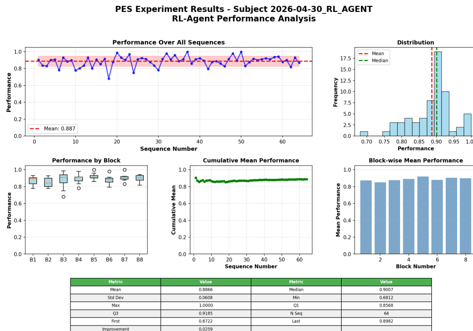
Figura 5.6: Desempeño por secuencia, distribución, estadísticos por bloque y resumen descriptivo de pes_q1.
