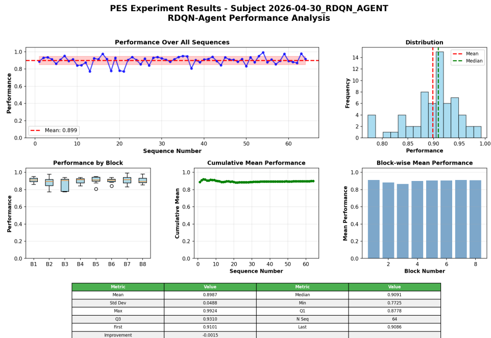
Figura 5.9: Desempeño por secuencia, distribución, estadísticos por bloque y resumen descriptivo de pes_rdn.
