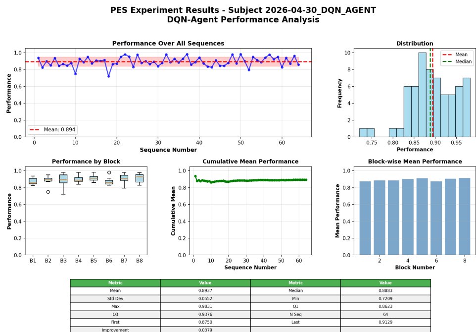
Figura 5.8: Desempeño por secuencia, distribución, estadísticos por bloque y resumen descriptivo de pes_dqn.
