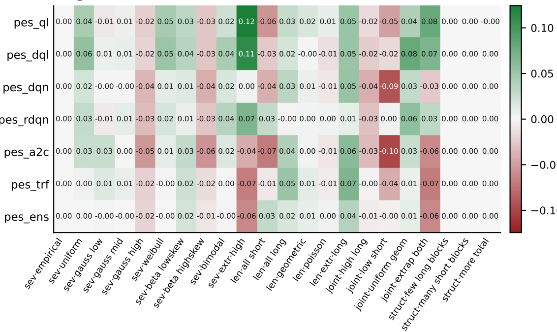
Degradación OOD \Delta r
