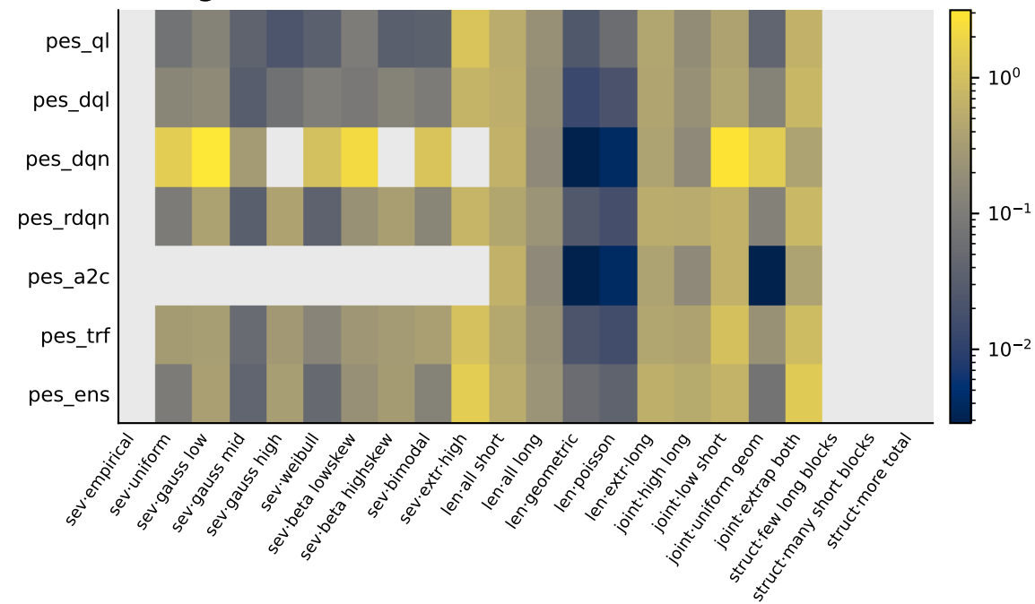
Divergencia KL de acciones
