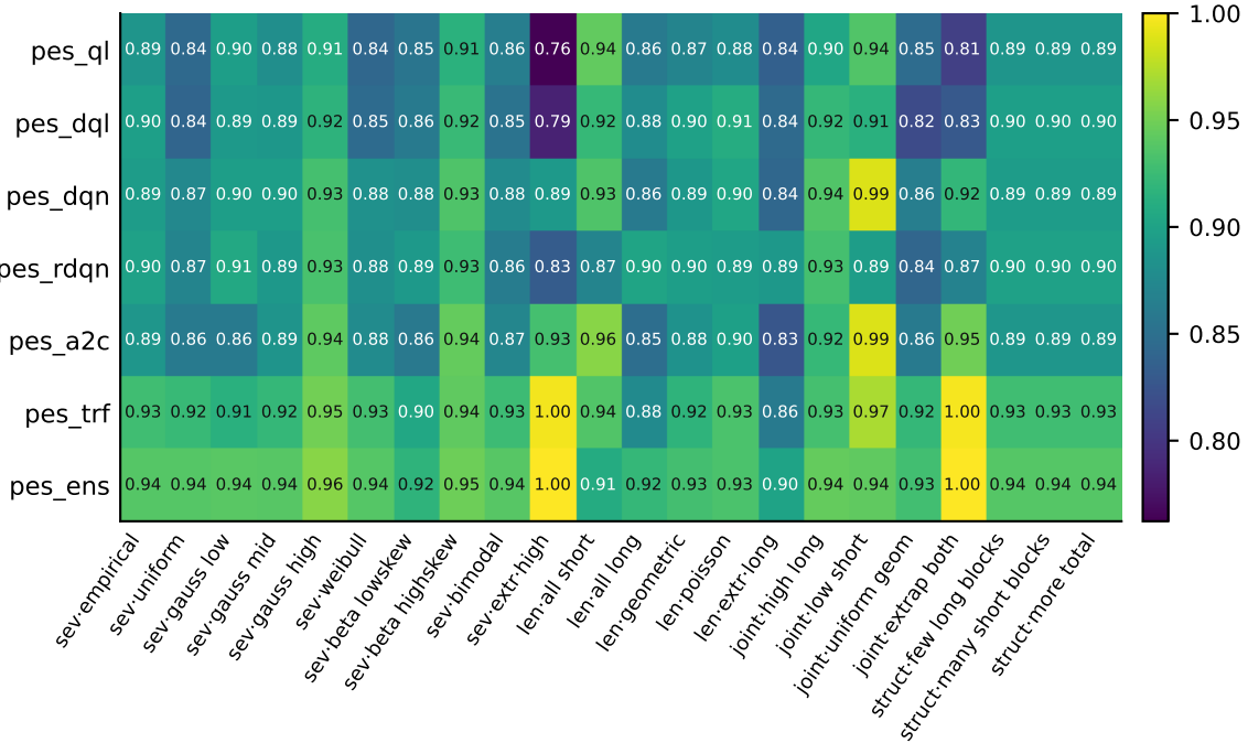
Retorno medio \bar{r}
