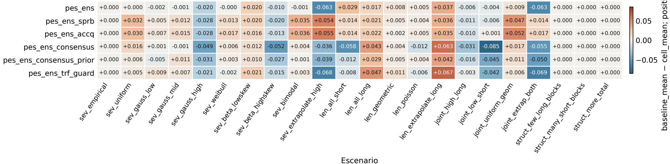
Ensemble: degradación respecto a sev_empirical
