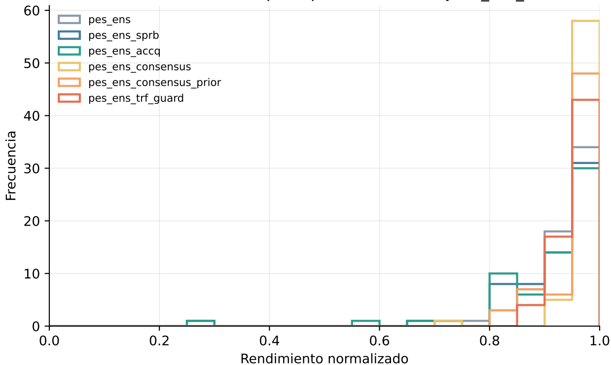
Distribución del desempeño por secuencia — joint_low_short
