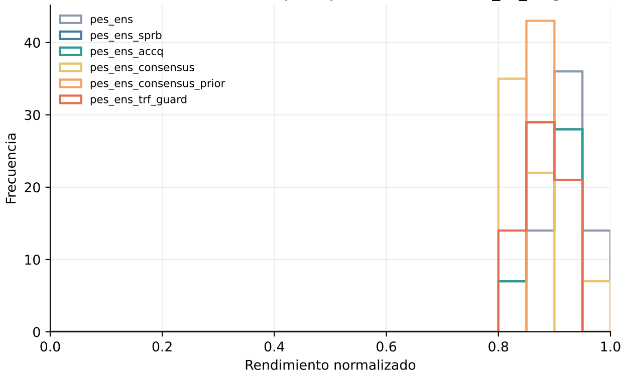
Distribución del desempeño por secuencia — len_all_long
