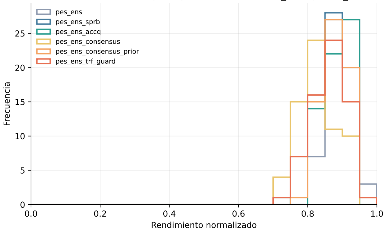
Distribución del desempeño por secuencia — len_extrapolate_long
