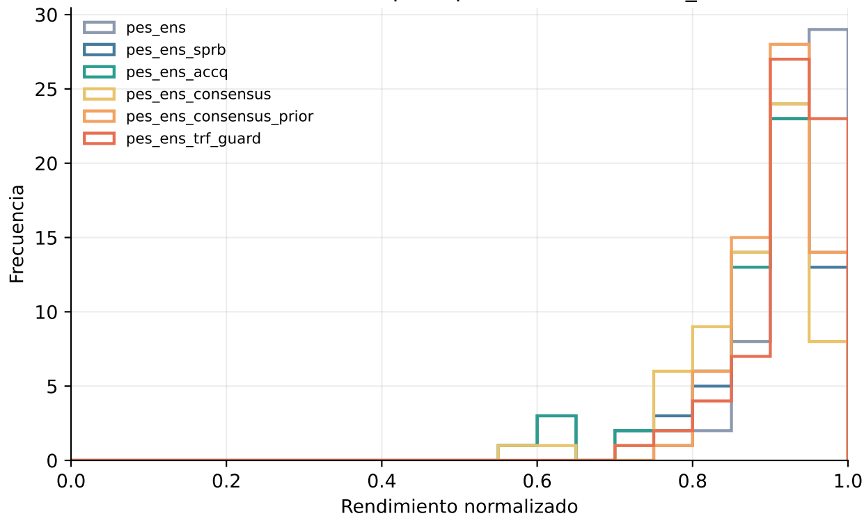
Distribución del desempeño por secuencia — sev_uniform
