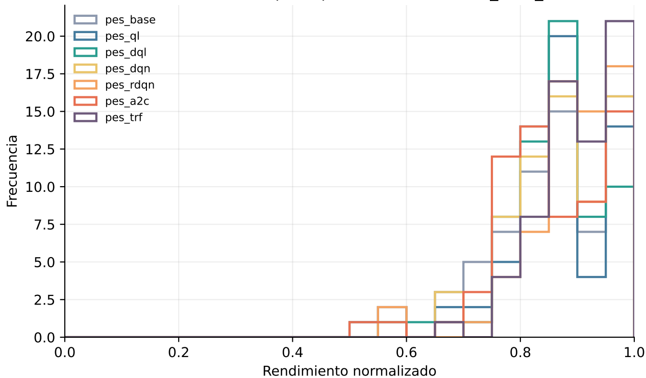
Distribución del desempeño por secuencia — sev_beta_lowskew
