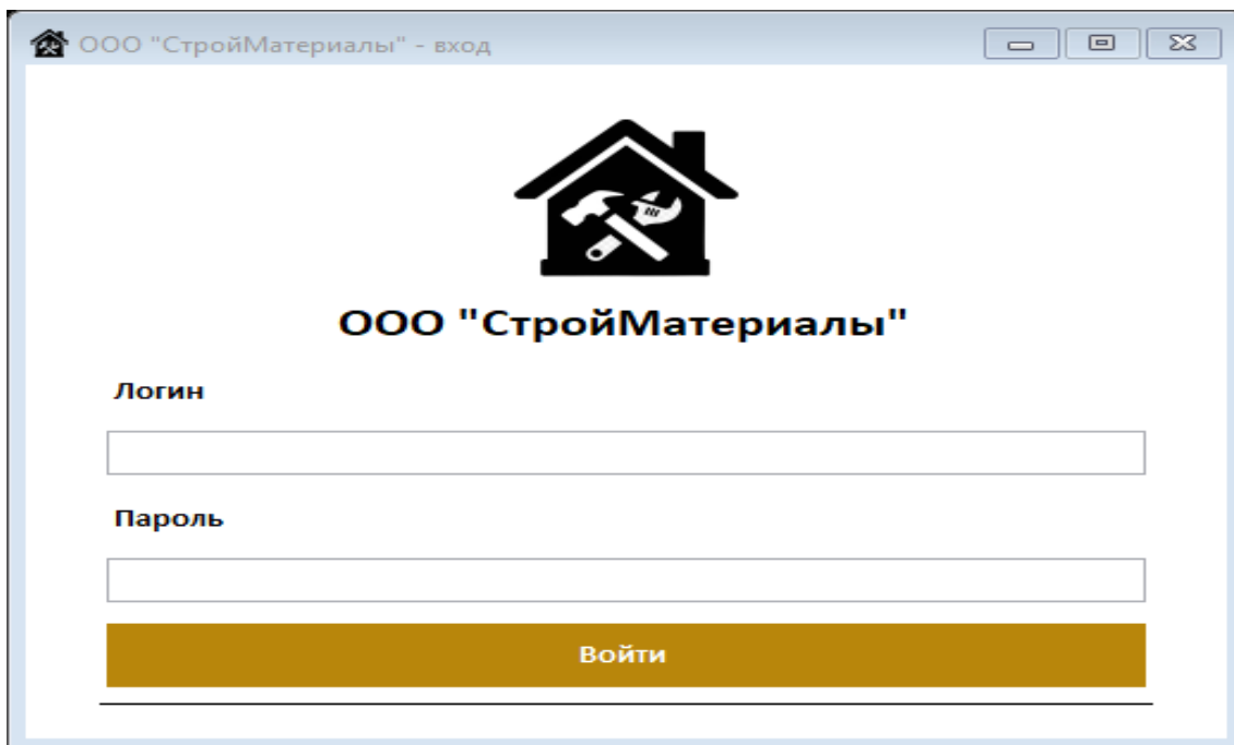
Рисунок 1 - Окно входа
