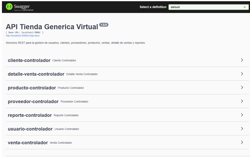
Figura 16. Documentación interactiva de la API generada con Swagger UI.
