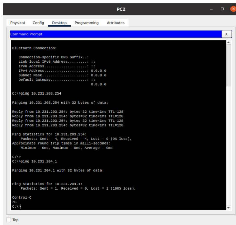
Рис. 3.4.9. Демонстрация доступа к компьютерам сети с PC2
