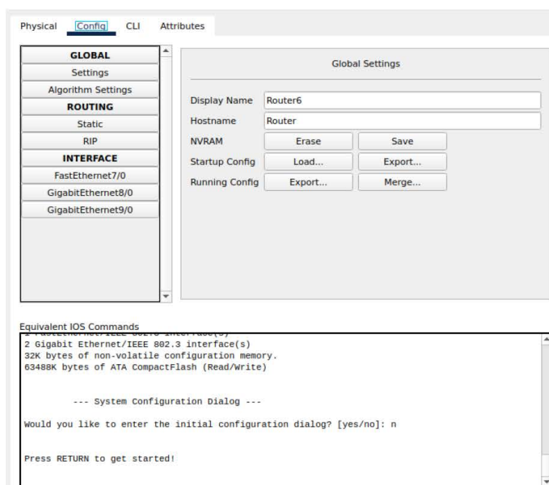
Рис. 7.4.4. Состав добавленных интерфейсов
