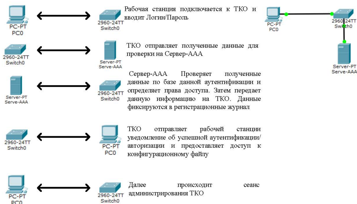
Рис. 4.3.2. Процесс внешней авторизации, аутентификации и учета
