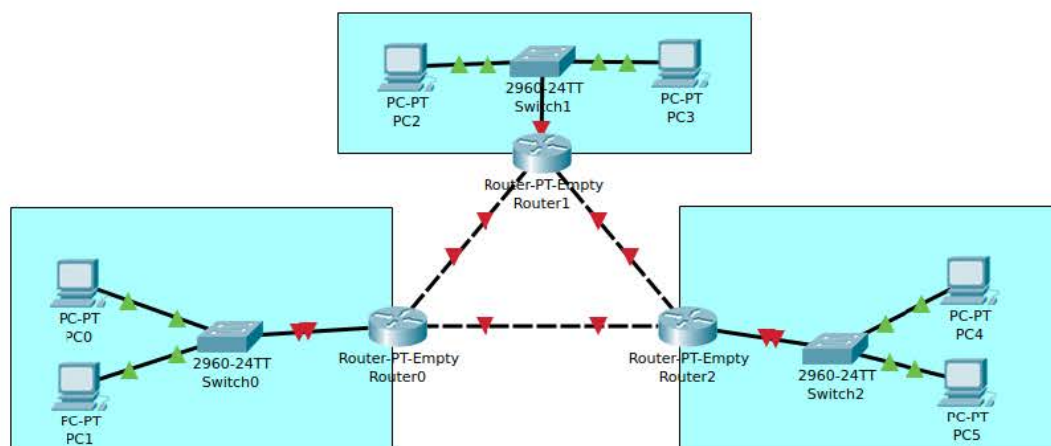
Рис. 7.4.1. Топология сети для практической работы
