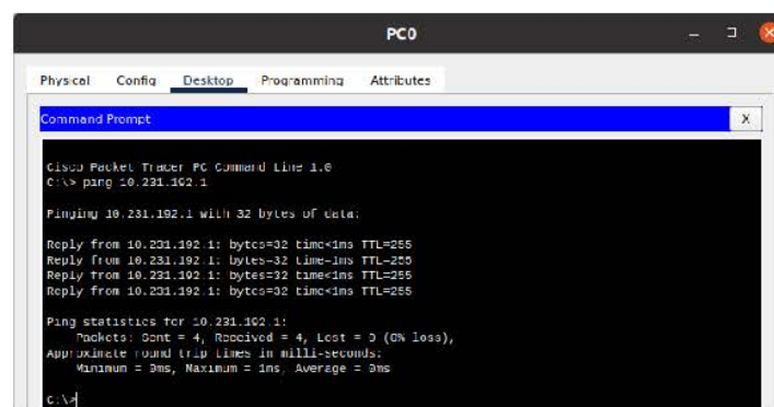
Рис. 7.4.7. Демонстрация доступа PC0 к Router0
