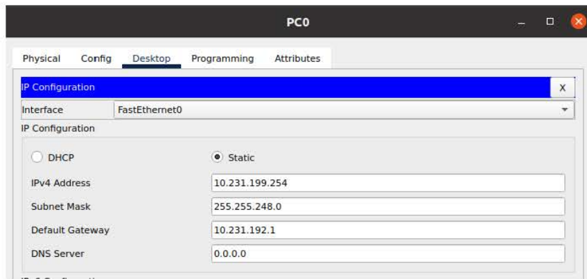
Рис. 7.4.6. Пример настройки PC0 для первой подсети
