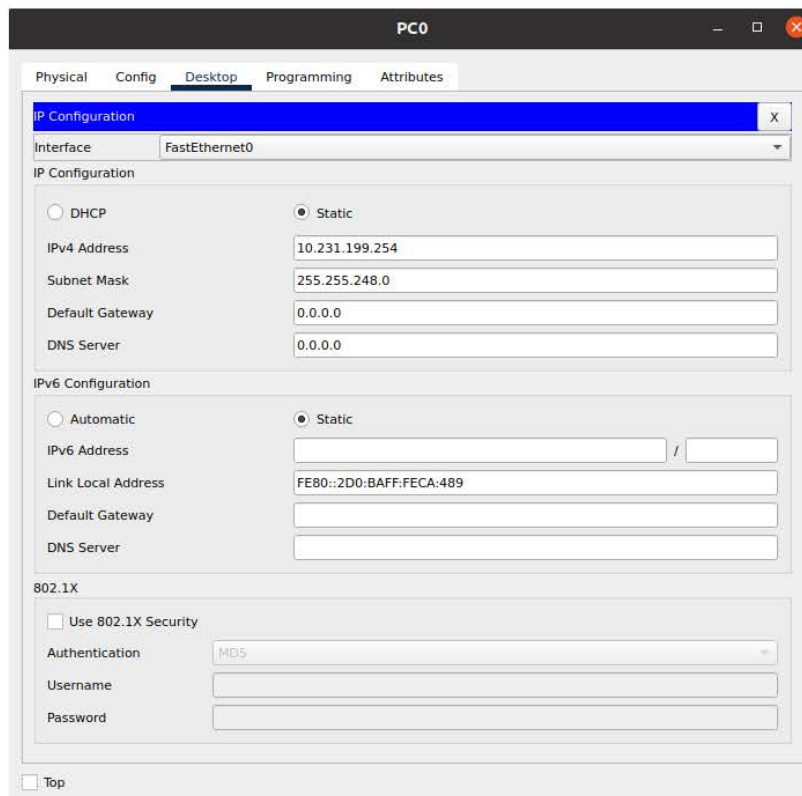
Рис. 3.4.7. Конфигурирование PC0
