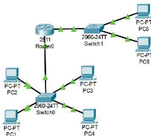
Рис. 2.4.6. Топология сети
