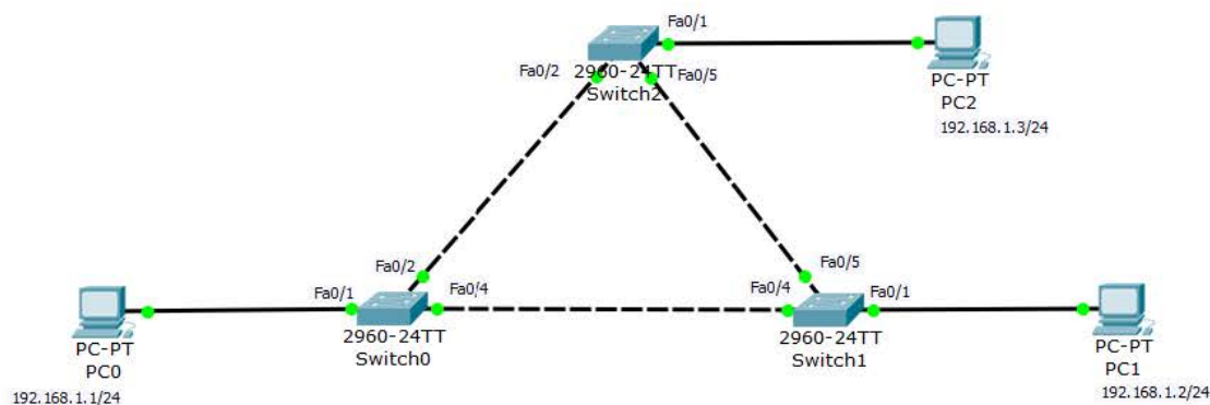
Рис. 9.4.1. Исходная топология сети
