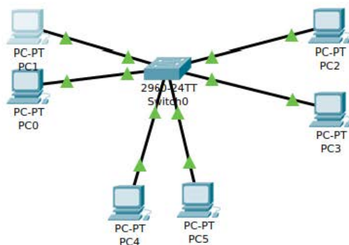
Рис. 3.4.6. Топология сети с использованием маски переменной длины
