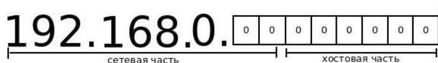
Рис. 3.3.1. Пример заимствования бит из хостовой части в сетевую
