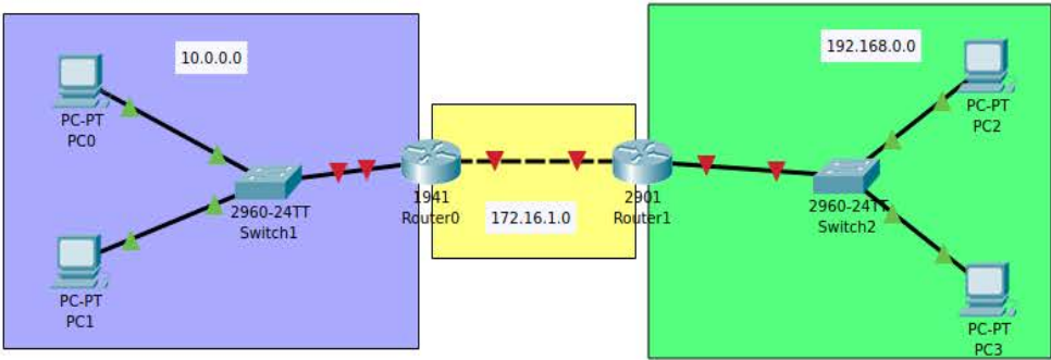
Рис. 7.3.11. Пример топологии сети для настройки статического маршрута
