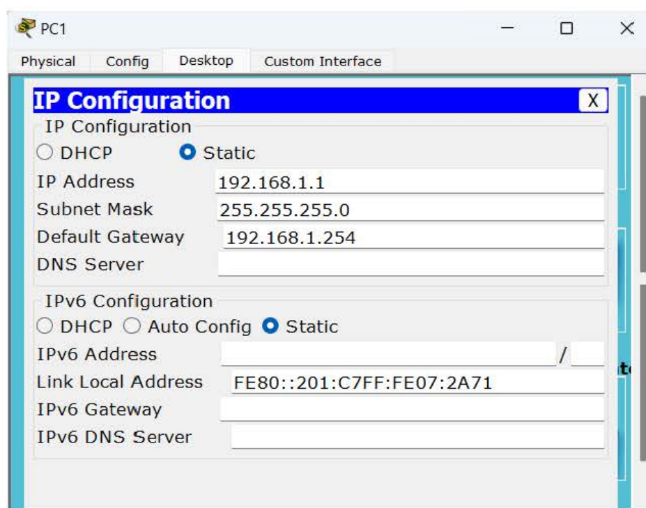
Рис. 2.4.7. Конфигурирование левого компьютера (PC1)
