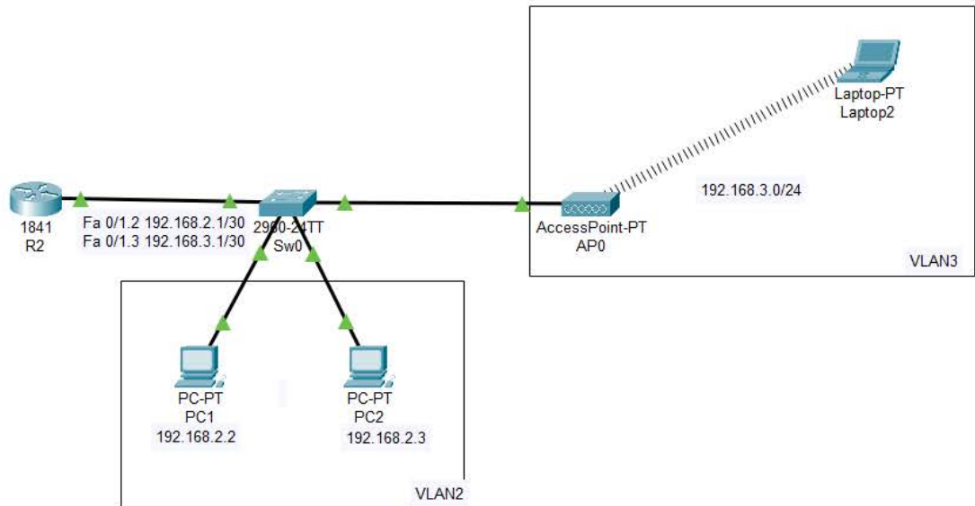
Рис. 10.4.3. Схема подключения беспроводной точки доступа
