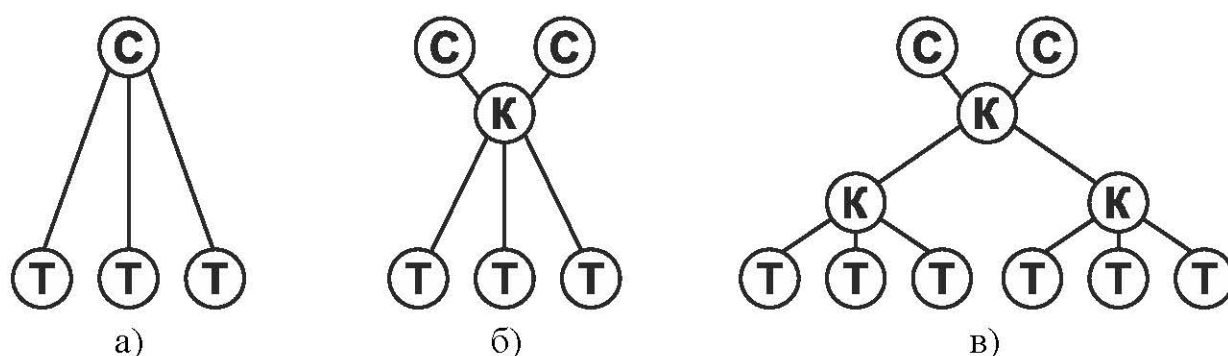
Рис. 5. Варианты реализации звездообразных структур: а) простейшая (одноуровневая); б) одноуровневая с использованием коммутатора; в) иерархическая звезда; Т — терминальное устройство; К — коммутатор; С — сервер
