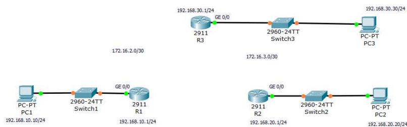
Рис. 8.4.1. Исходная топология сети
