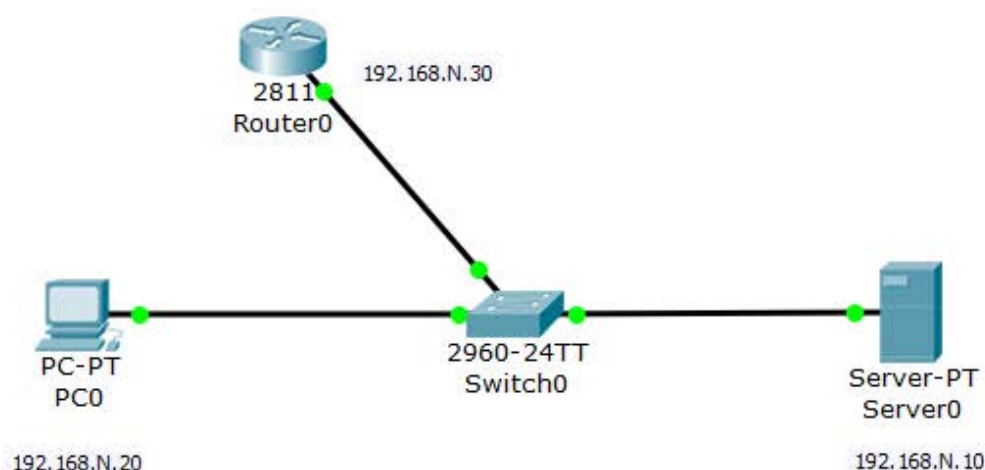
Рис. 5.4.1. Схема моделируемой сети
