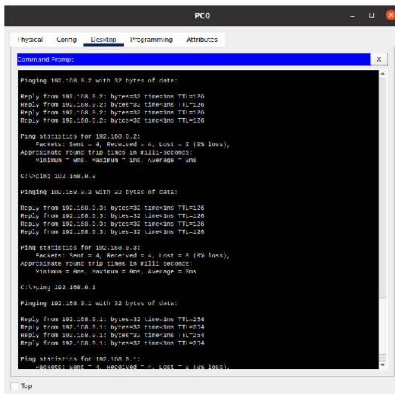
Рис. 7.3.23. Проверка доступа к сети 192.168.0.0 из сети 10.0.0.0
