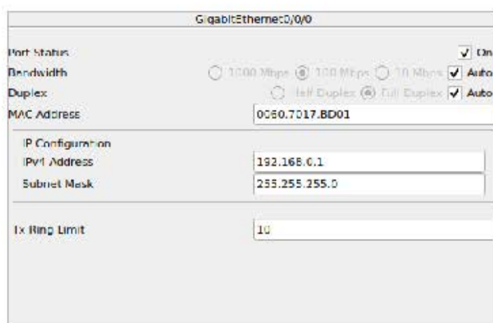
Рис. 7.3.2. Конфигурирование интерфейса GigabitEthernet 0/0/0 роутера
