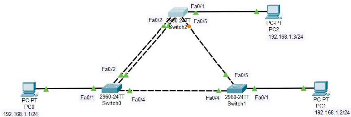
Рис. 9.4.2. Агрегация канала между Switch0 и Switch2
