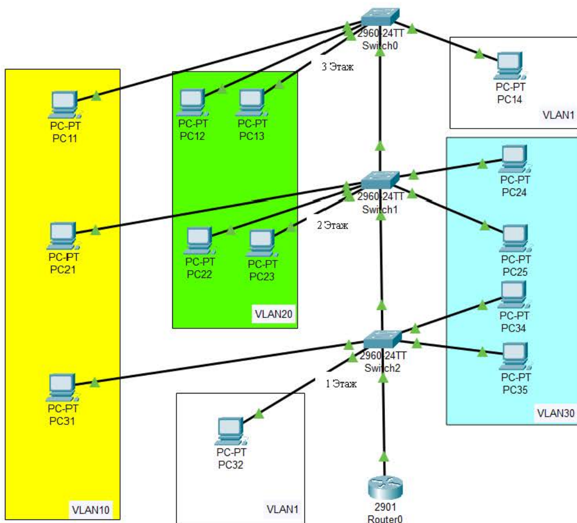
Рис. 6.4.6. Топология сети с дополнительным маршрутизатором
