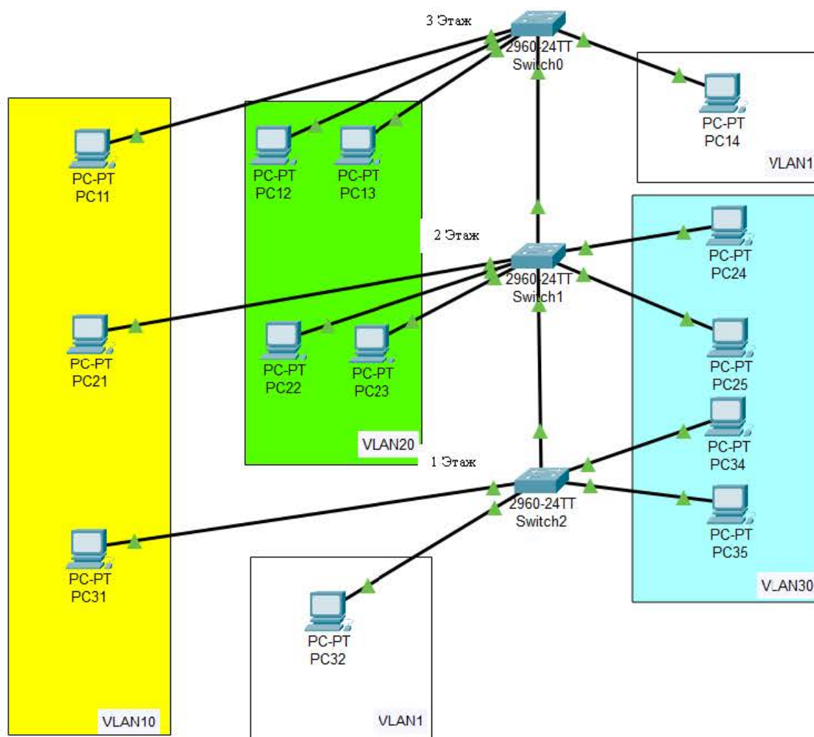
Рис. 6.4.1. Топология сети
