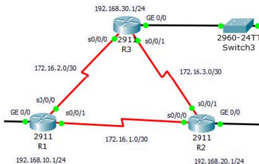
Рис. 8.4.3. Схема подключения маршрутизаторов
