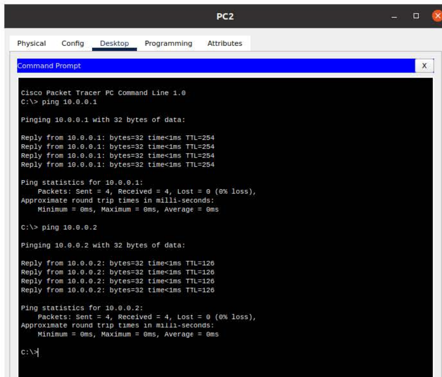
Рис. 7.3.24. Проверка доступа к сети 10.0.0.0 из сети 192.168.0.0
