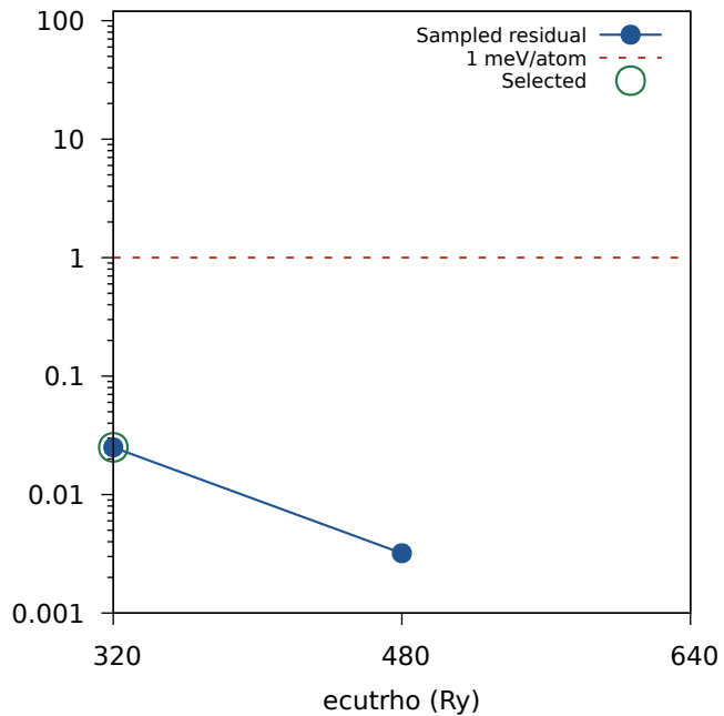
(b) ecutrho
