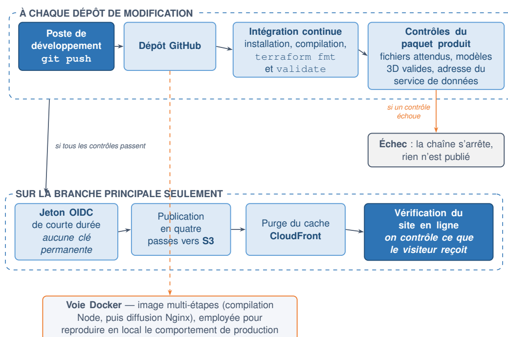
FIGURE 3.5 : Chaîne d'intégration et de déploiement continu en service
