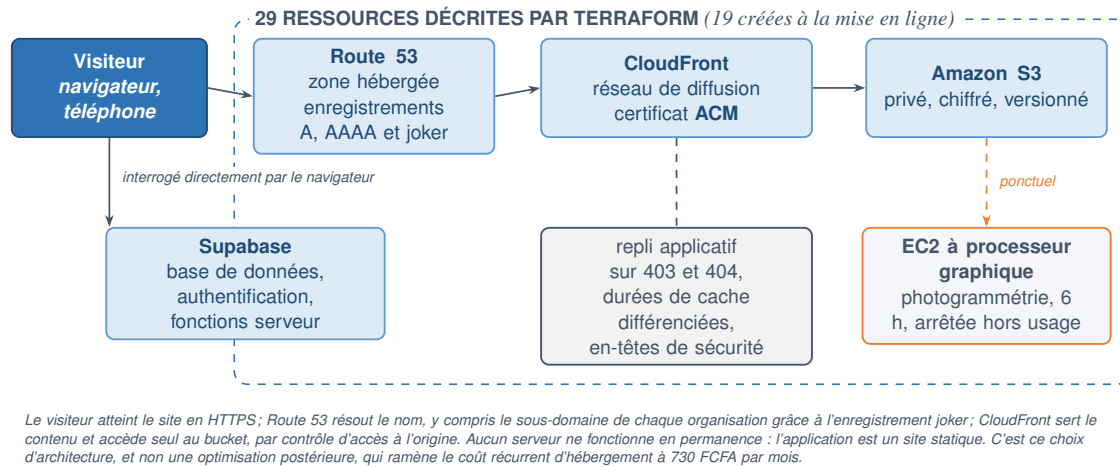
FIGURE 3.4 : Architecture de l'infrastructure d'hébergement en nuage
