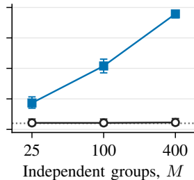
(d) Fixed peers Opposed effects
