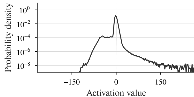
(e) Logits
