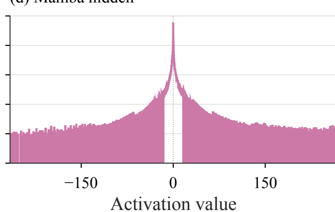
(d) Mamba hidden
