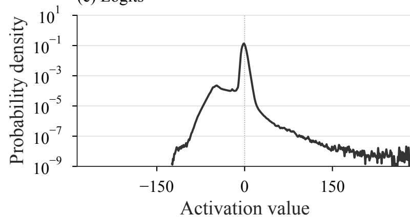
(e) Logits
