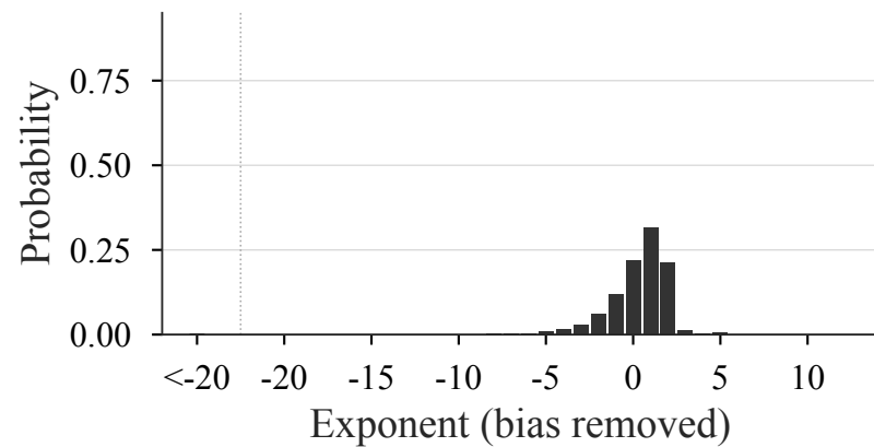
(e) Logits
