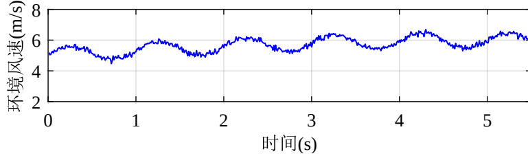
图 3-3 模拟环境风速扰动结果
