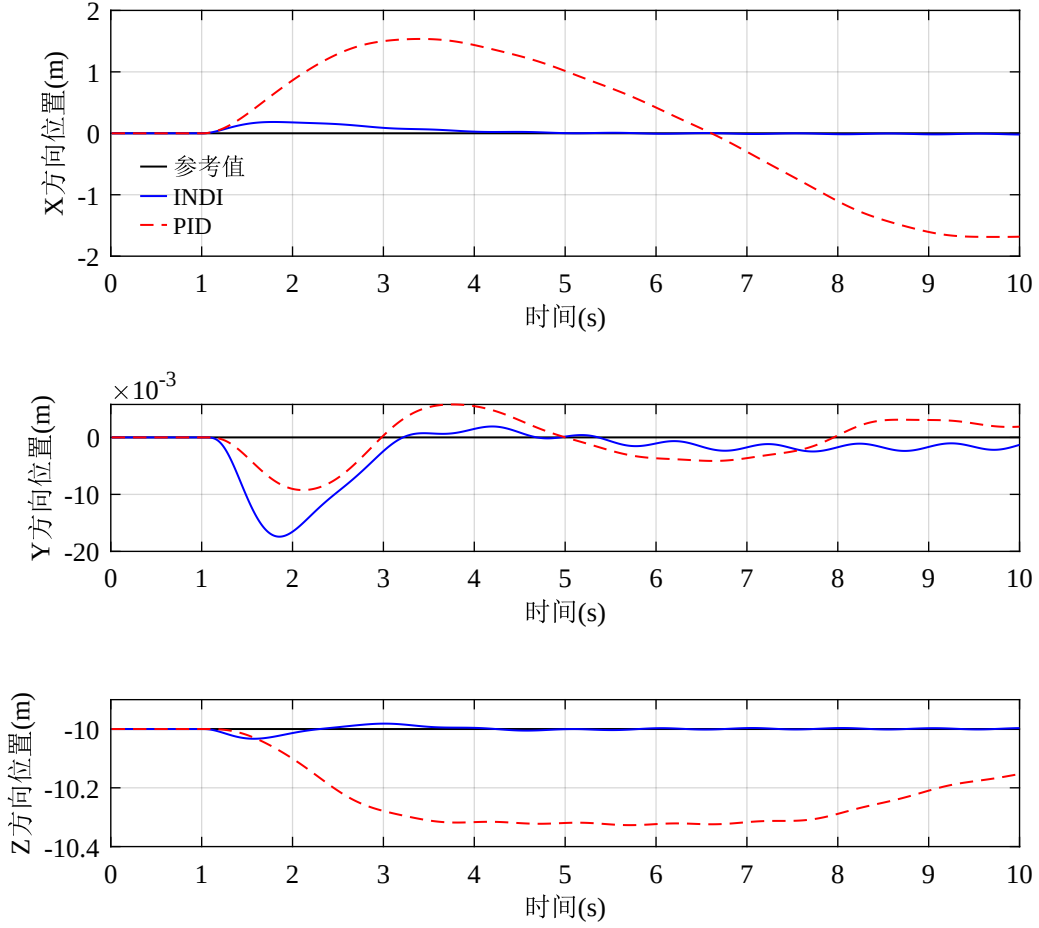
图 3-4 INDI 位置控制定点悬停抗风实验仿真结果
