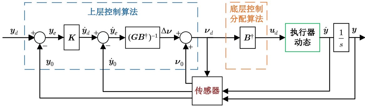
图 3-1 INDI 控制律的求逆操作表示为增量控制分配问题示意框图
