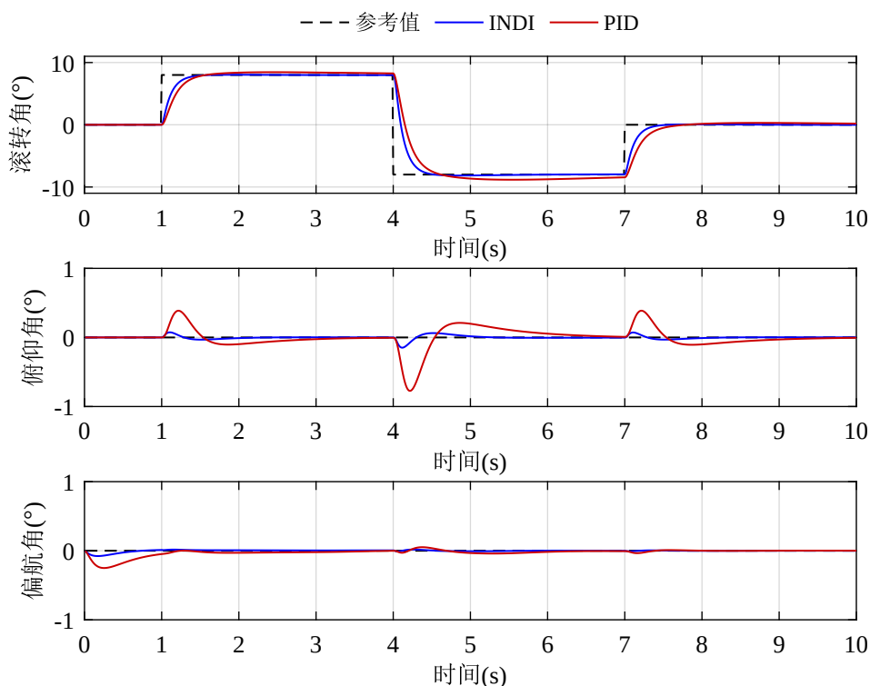
图 3-4 INDI 对比 PID 在无扰动情况下的仿真实验结果
