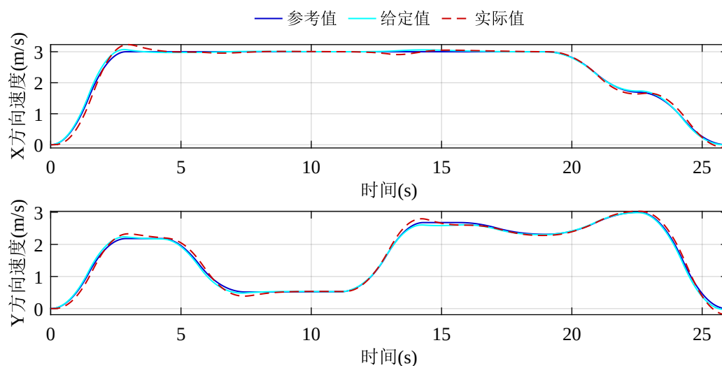
图 5-15 速度曲线规划与跟踪结果
