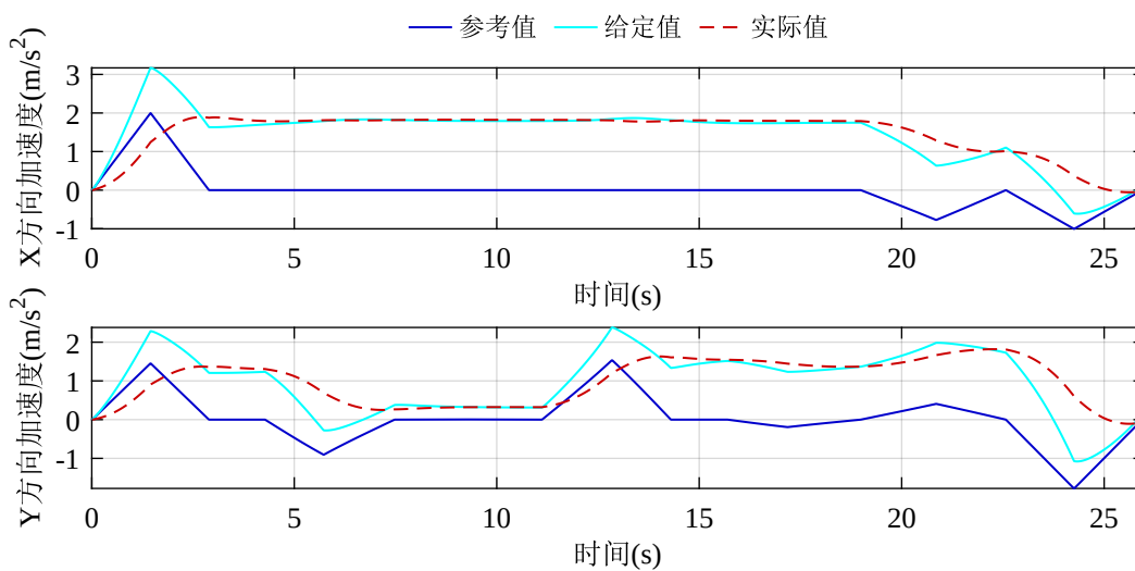
图 5-16 加速度曲线规划与跟踪结果
