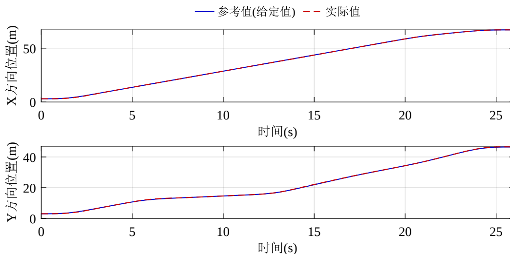
图 5-14 位置曲线规划与跟踪结果
