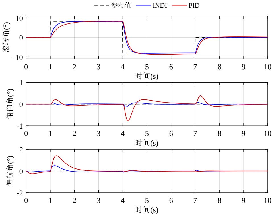
图 3-5 INDI 对比 PID 在有扰动情况下的仿真实验结果
