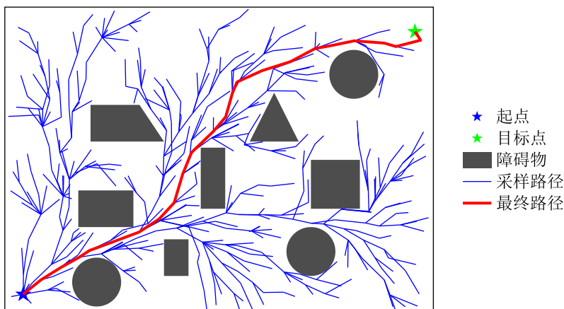
图 5-3 RRT* 算法随机树生成示意图
