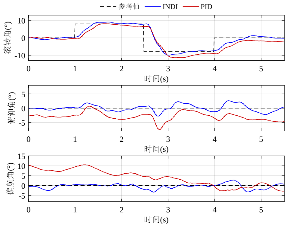
图 3-11 INDY 对比 PID 有扰动时的飞行试验结果
