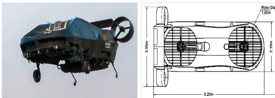
a) AirMule 无人机
