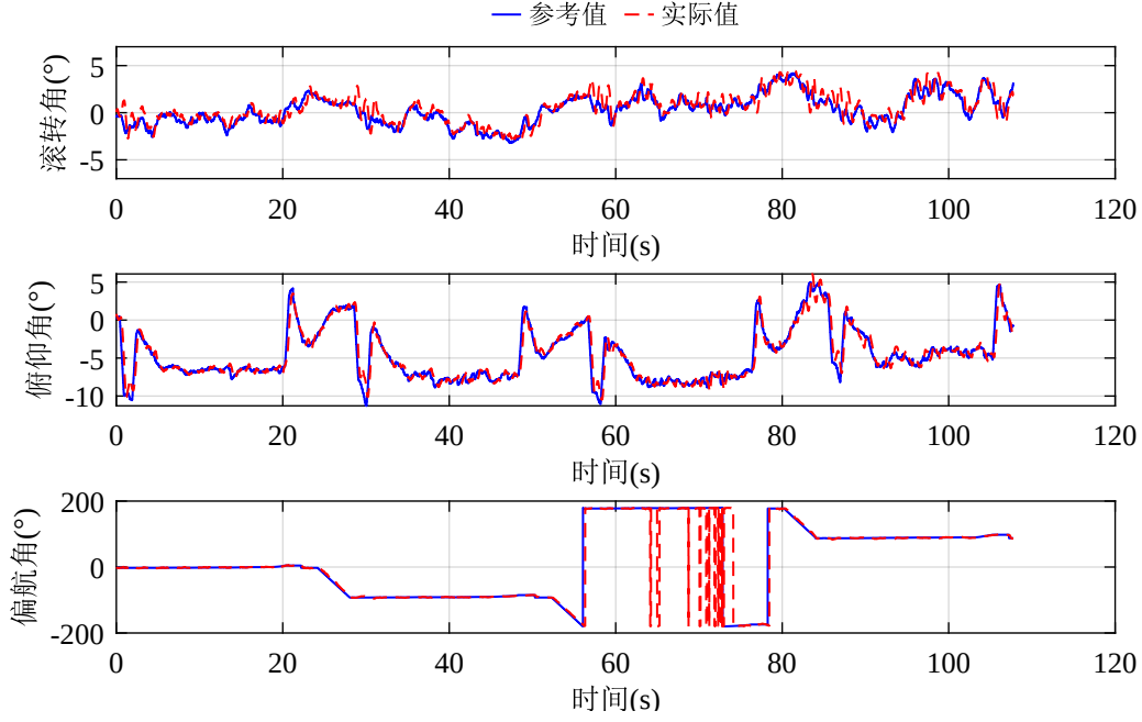
图 4-8 点对点轨迹飞行实验姿态跟踪结果
