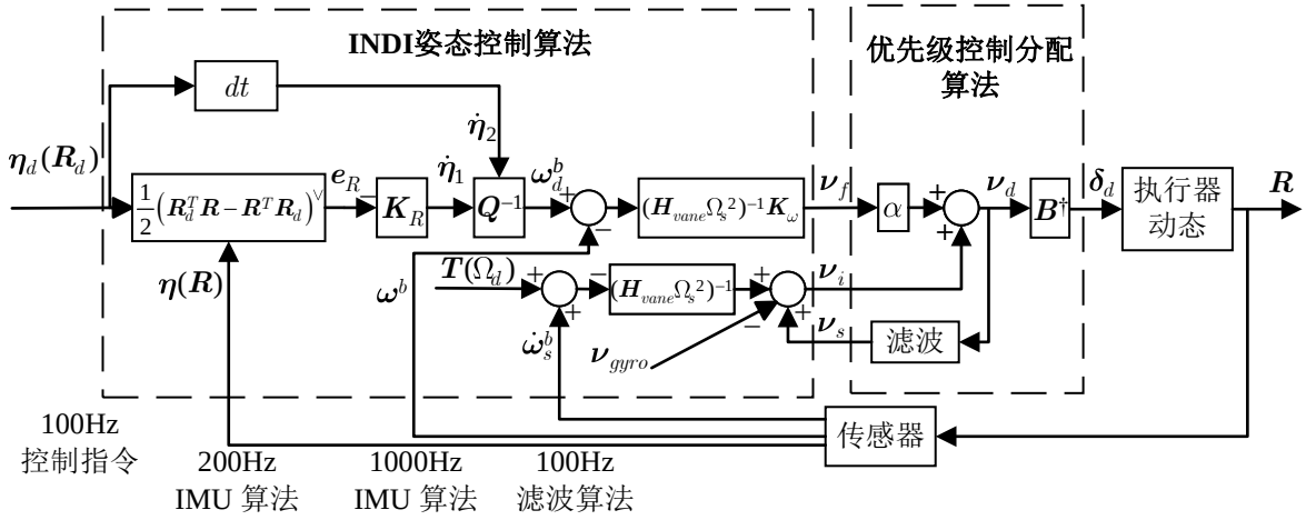
图 3-2 基于 INDI 和优先级控制分配法的姿态控制系统框图
