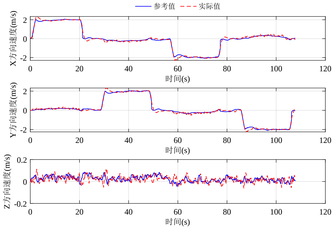
图 4-8 点对点轨迹飞行试验速度跟踪结果
