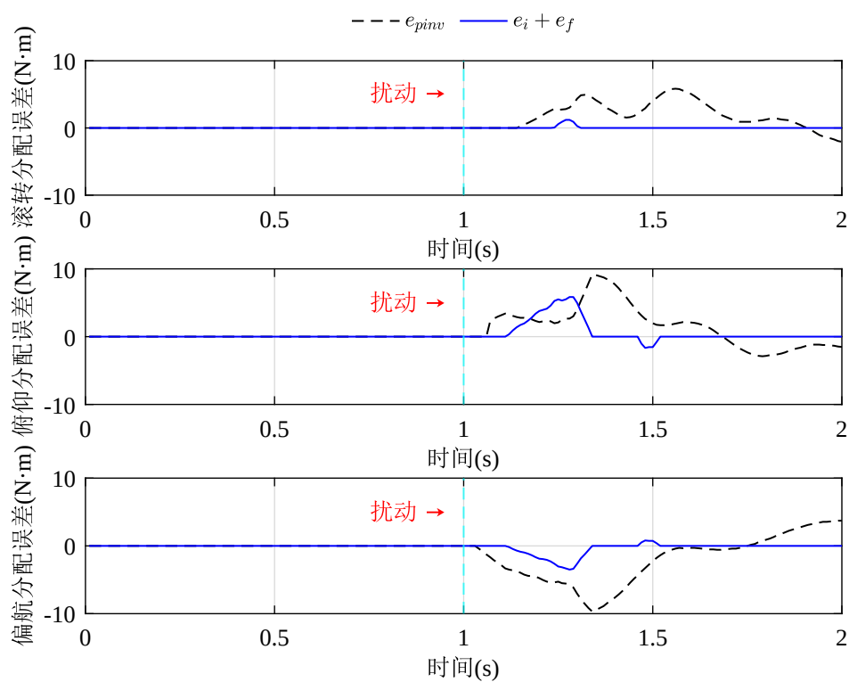
图 3-13 优先级对比伪逆的分配误差飞行试验结果
