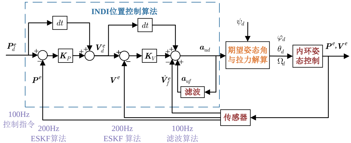
图 4-2 INDI 位置控制系统框图
