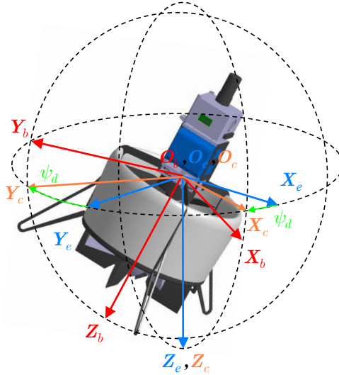
图 4-1 中间坐标系示意图
