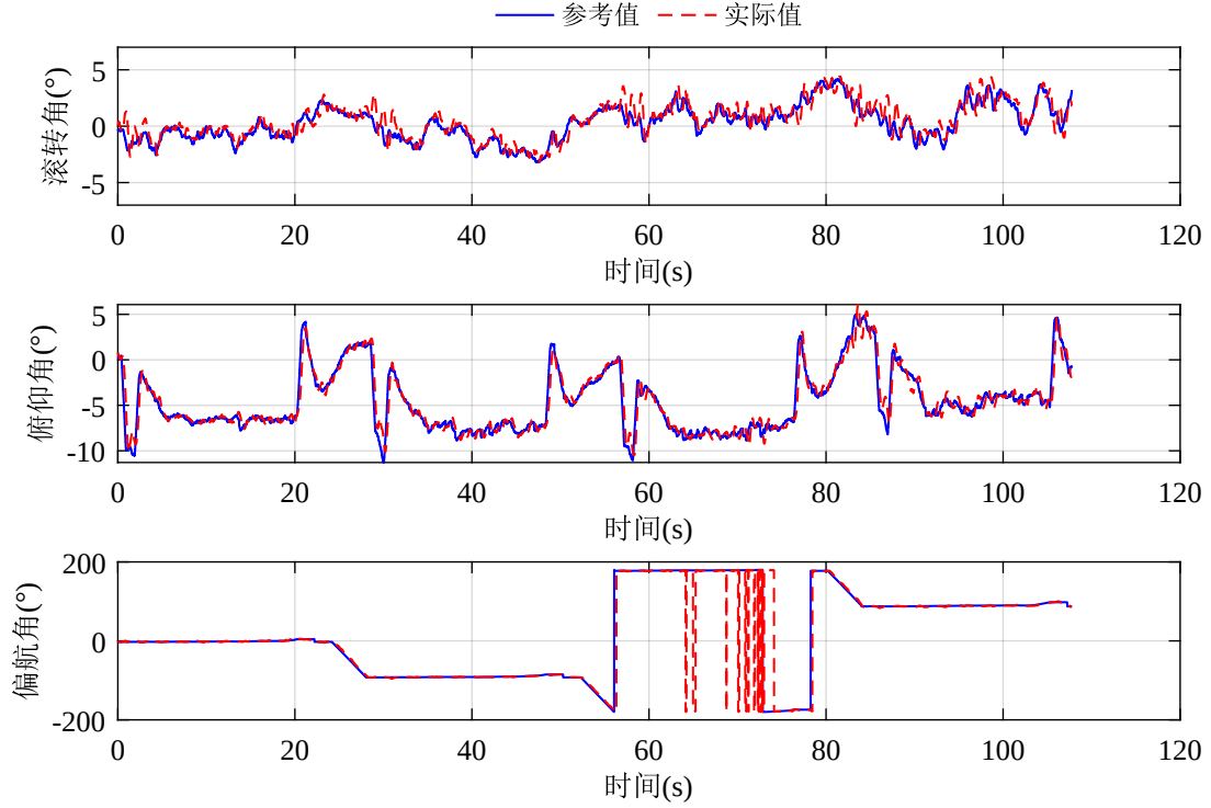
图 4-9 点对点轨迹飞行试验姿态跟踪结果
