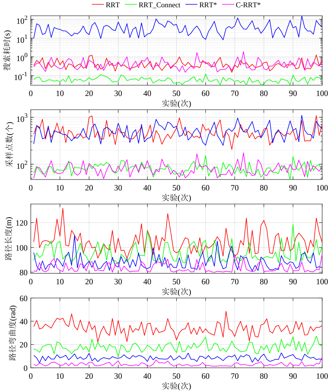
图 5-11 高密度障碍物下四种算法性能对比
