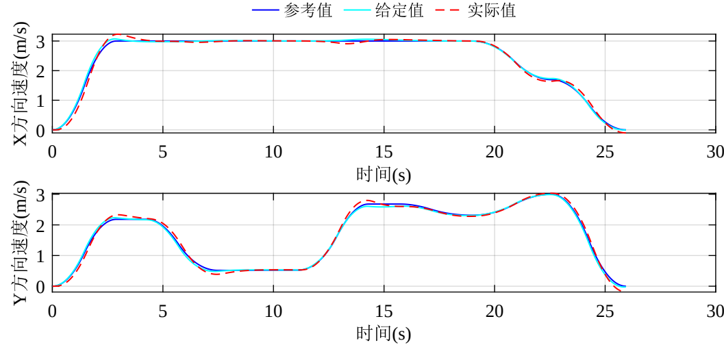
图 5-15 速度曲线规划与跟踪结果
