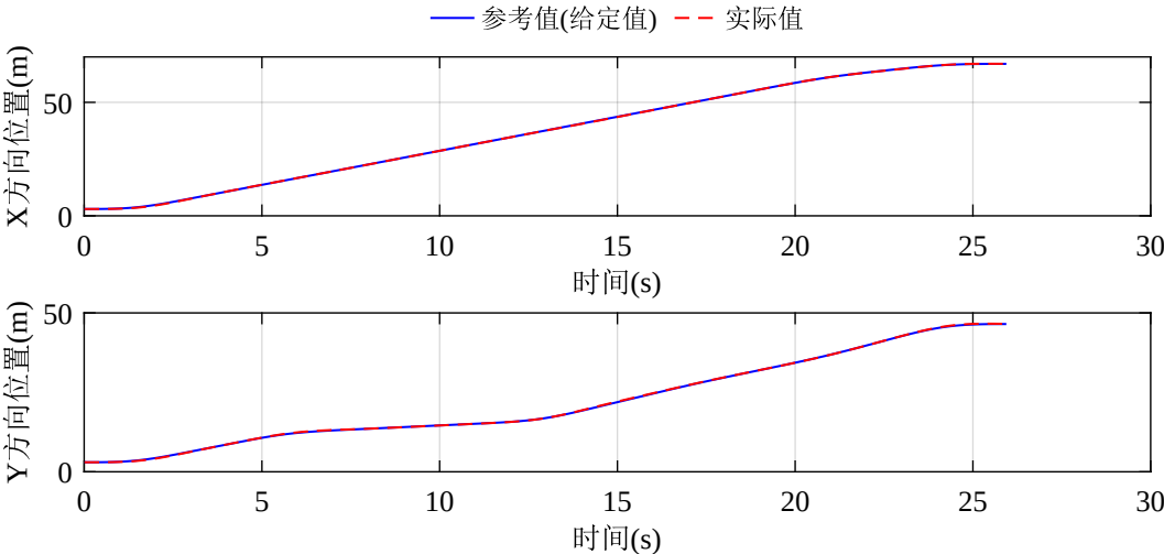
图 5-14 位置曲线规划与跟踪结果
