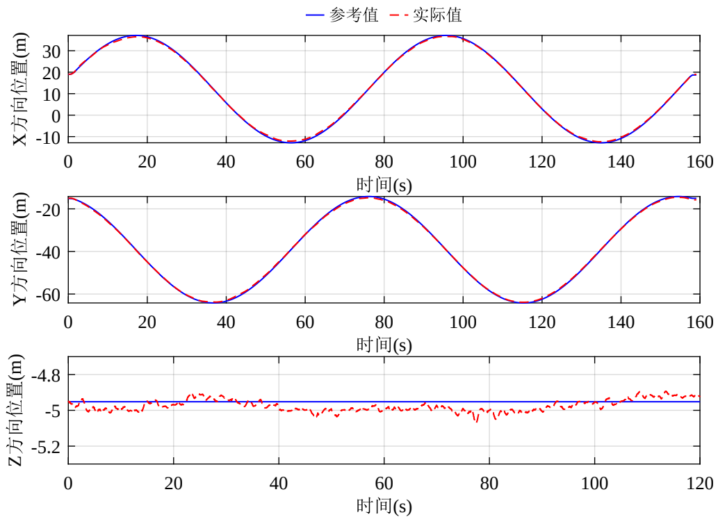
图 3-10 圆弧轨迹飞行实验位置跟踪结果
