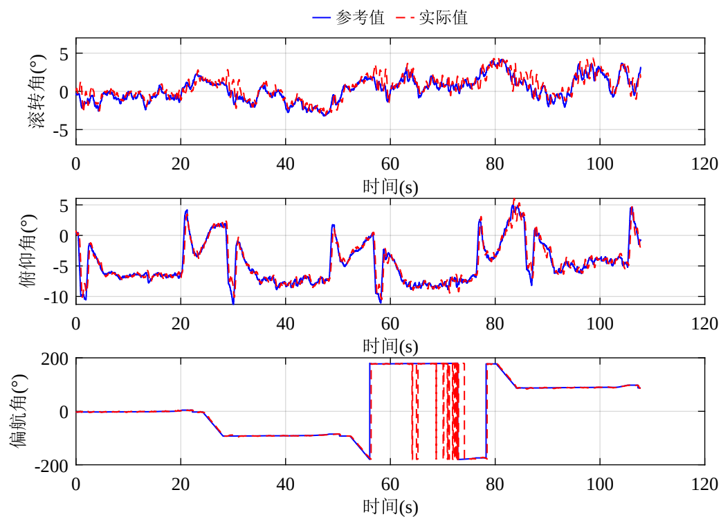
图 3-8 点对点轨迹飞行实验姿态跟踪结果
