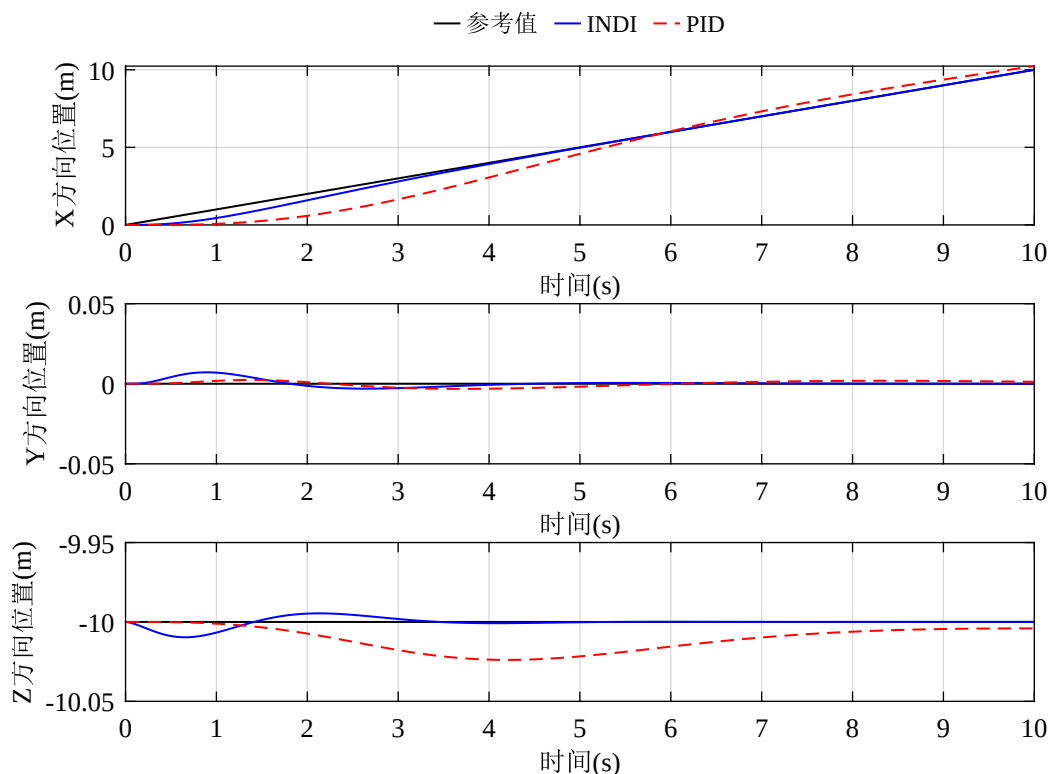
图 3-5 INDI 对比 PID 位置控制轨迹跟踪实验仿真结果
