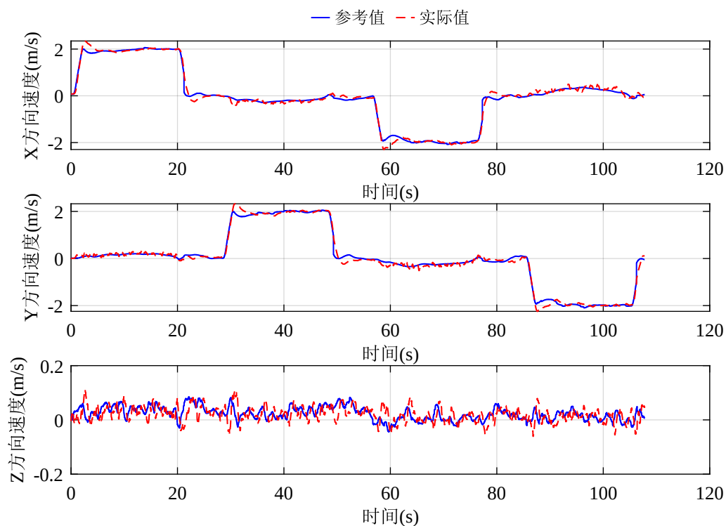
图 3-7 点对点轨迹飞行实验速度跟踪结果
