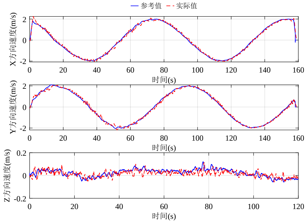
图 3-11 圆弧轨迹飞行实验速度跟踪结果
