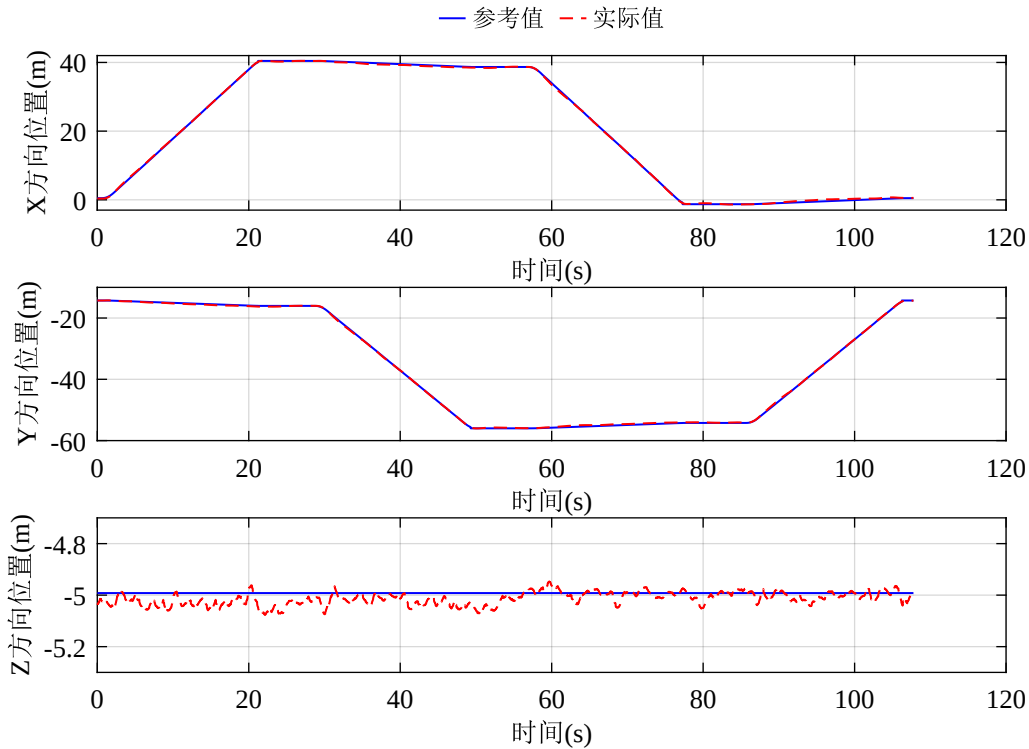
图 3-6 点对点轨迹飞行实验位置跟踪结果
