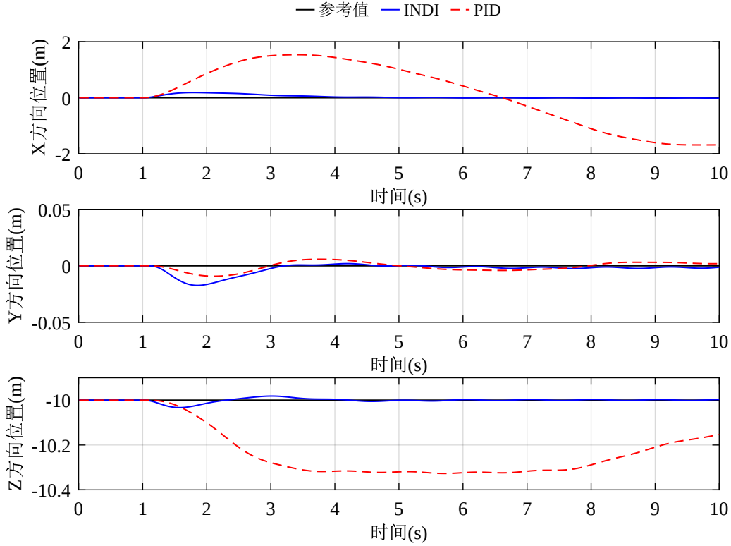
图 3-4 INDI 对比 PID 位置控制定点悬停抗风实验仿真结果
