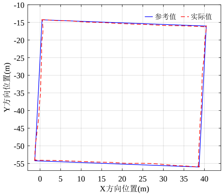
图 3-9 点对点轨迹飞行实验二维平面轨迹结果
