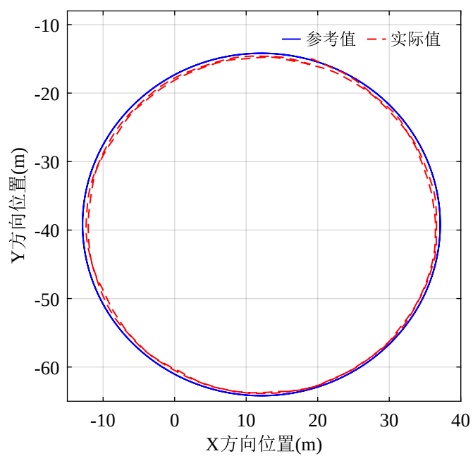
图 3-13 圆弧轨迹飞行实验二维平面轨迹结果
