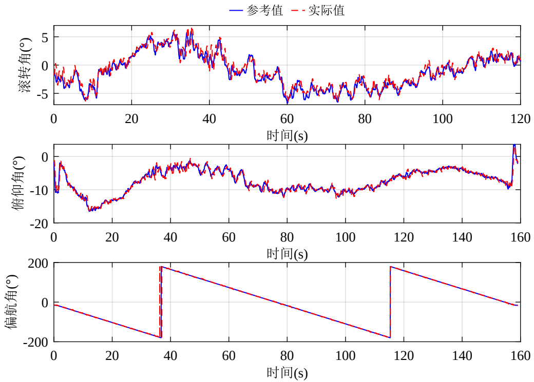
图 3-12 圆弧轨迹飞行实验姿态跟踪结果
