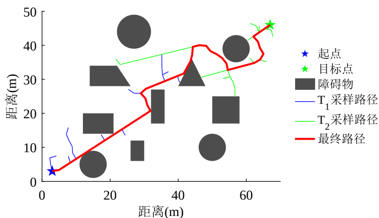
图 3-2 RRT-Connect 算法仿真实验结果
