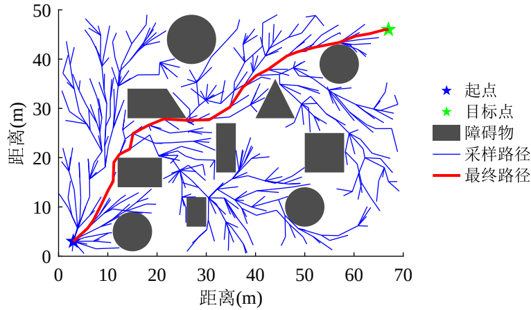
图 3-1 RRT 算法仿真实验结果
