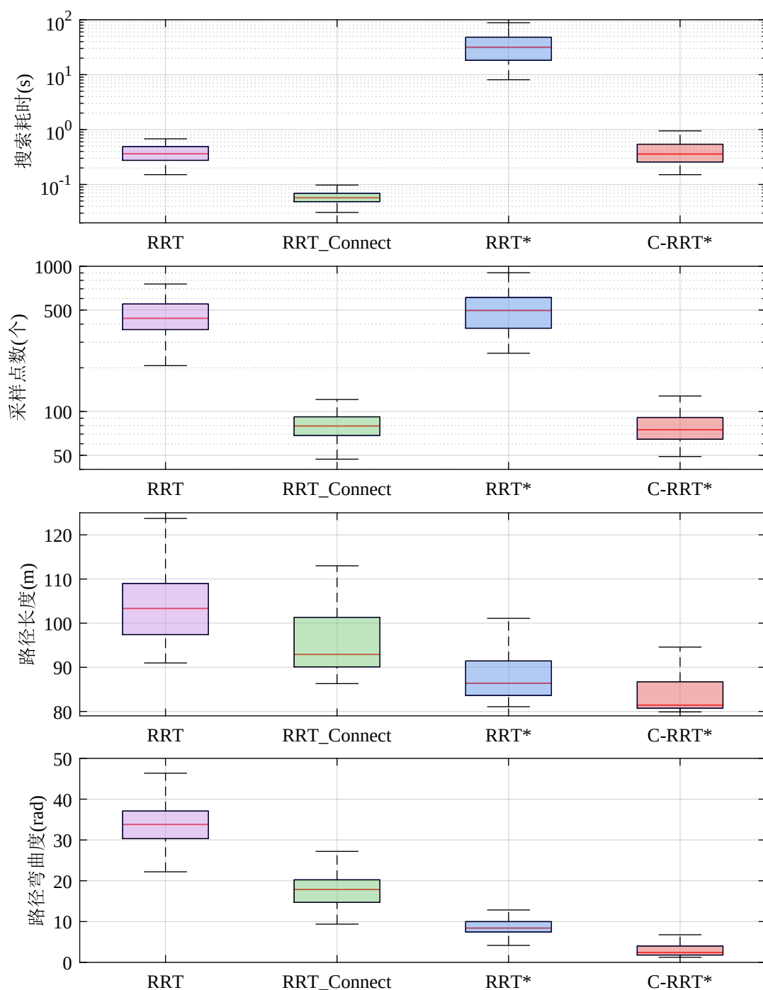
图 5-11 高密度障碍物下四种算法性能对比
