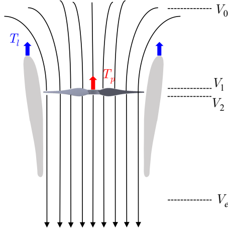
图 2-4 轴流状态的气动分析示意图
