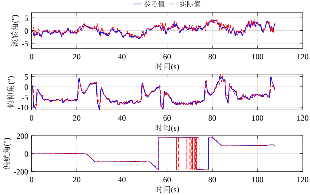
图 4-8 点对点轨迹飞行实验姿态跟踪结果
