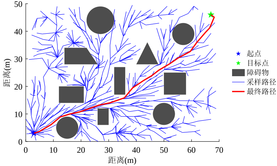
图 5-3 RRT* 算法仿真实验结果
