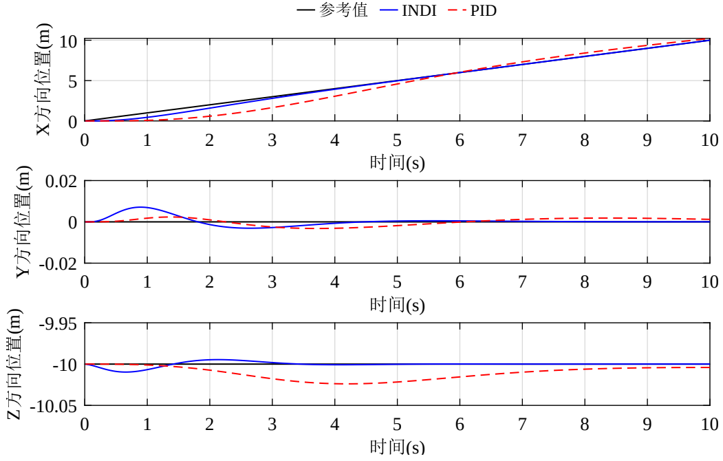
图 4-5 INDI 对比 PID 位置控制轨迹跟踪实验仿真结果
