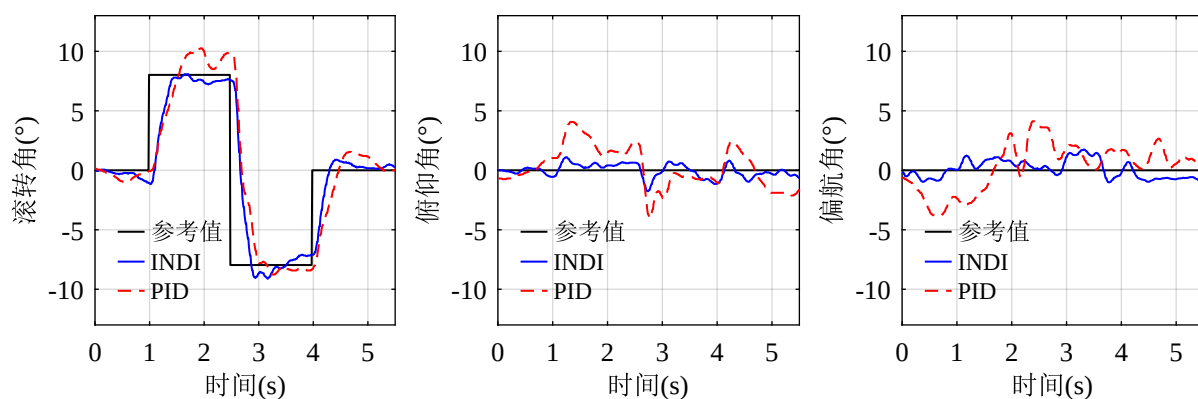
图 3-9 INDI 对比 PID 无扰动时的飞行实验结果
