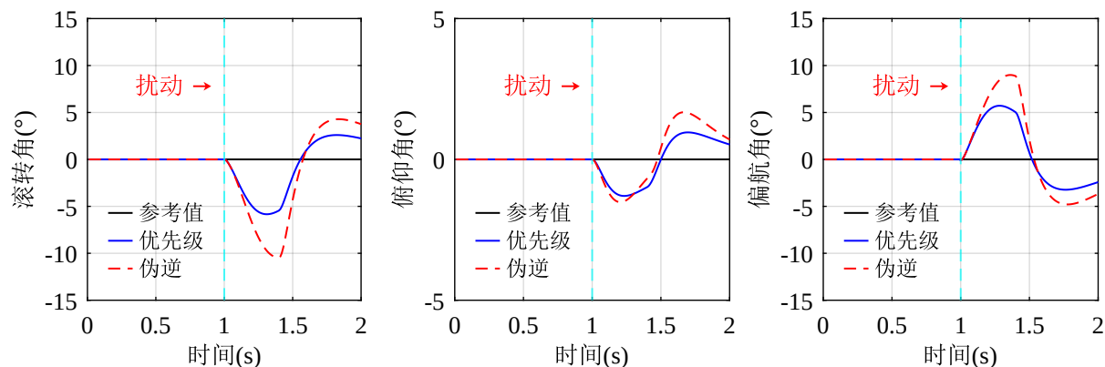
图 3-6 优先级控制分配对比伪逆法的姿态保持仿真实验结果
