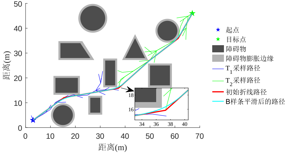
图 5-10 B 样条曲线路径平滑实验结果
