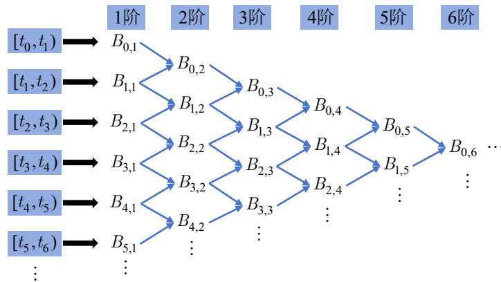
图 5-6 B 样条基函数递推关系示意图
