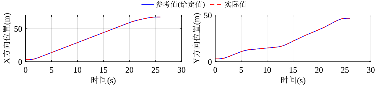
图 5-11 位置曲线规划与跟踪结果
