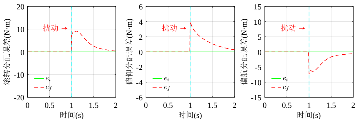
图 3-8 优先级分量各自的分配误差仿真实验结果
