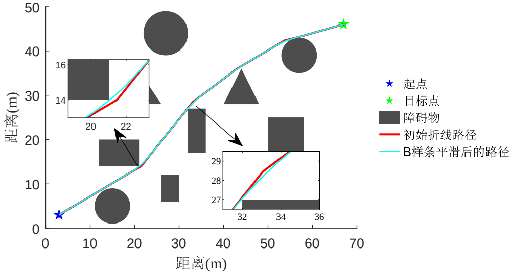
图 5-8 B 样条曲线路径平滑结果
