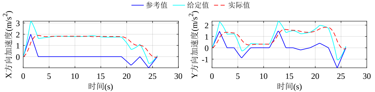
图 5-13 加速度曲线规划与跟踪结果
