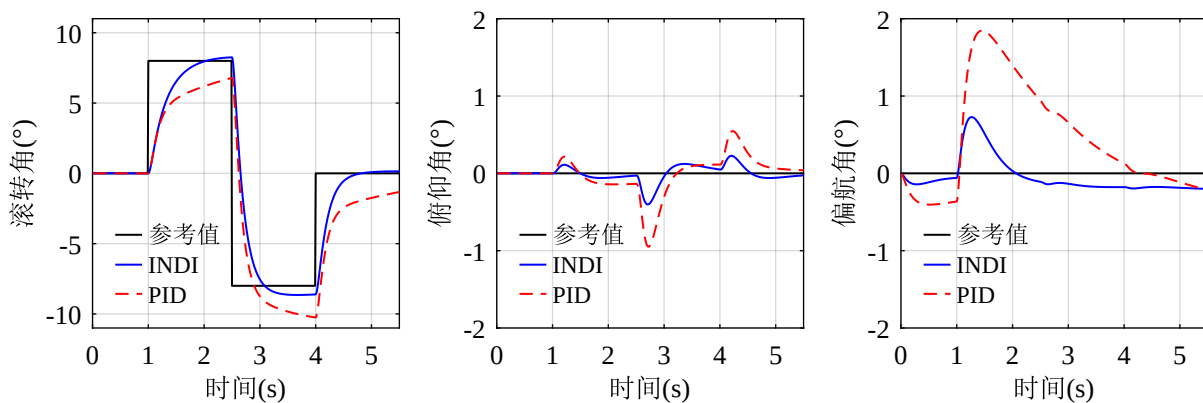
图 3-5 INDI 对比 PID 在有扰动情况下的仿真实验结果
