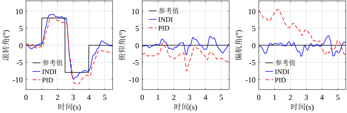
图 3-10 INDI 对比 PID 有扰动时的飞行实验结果
