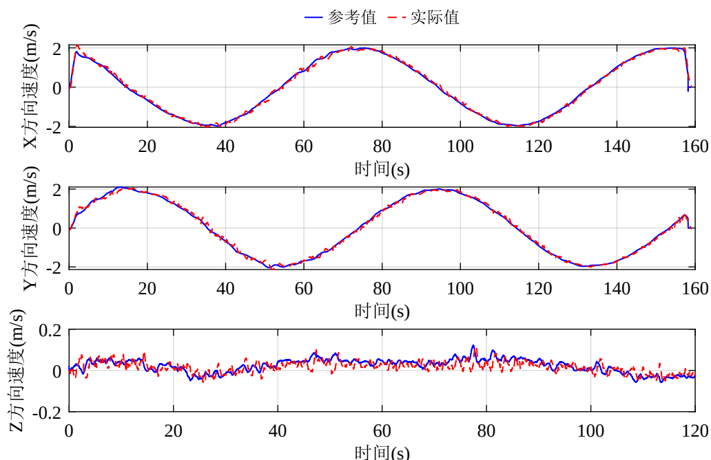
图 4-11 圆弧轨迹飞行实验速度跟踪结果
