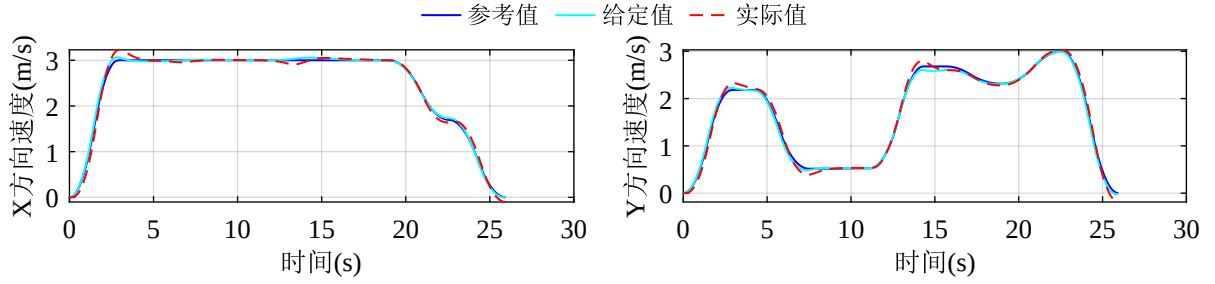
图 5-12 速度曲线规划与跟踪结果
