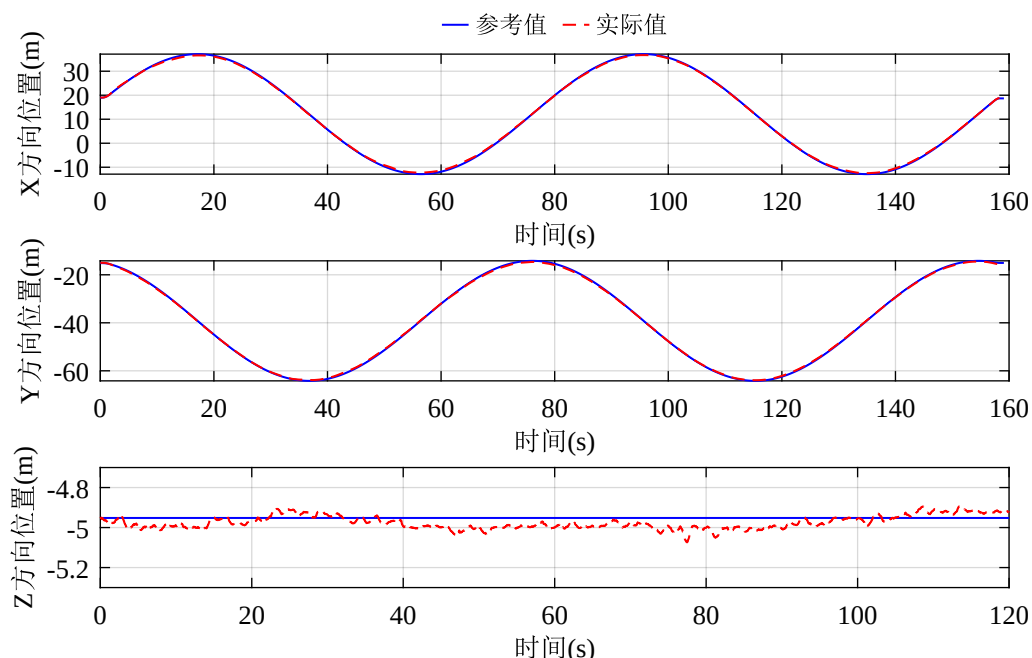
图 4-10 圆弧轨迹飞行实验位置跟踪结果
