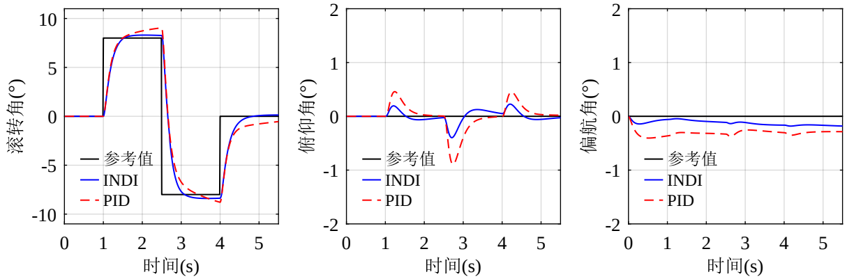
图 3-4 INDI 对比 PID 在无扰动情况下的仿真实验结果
