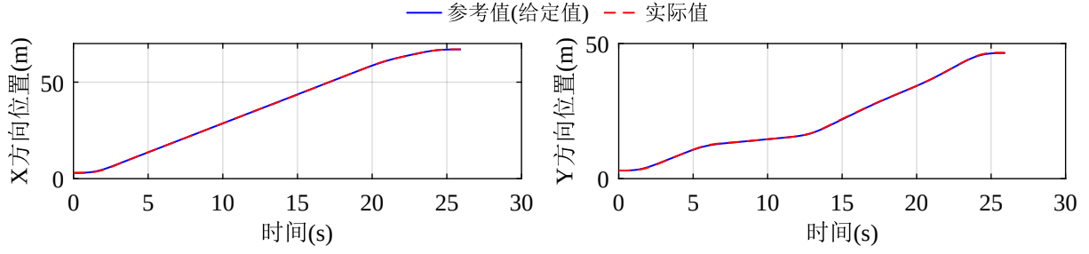
图 3-11 位置曲线规划与跟踪结果
