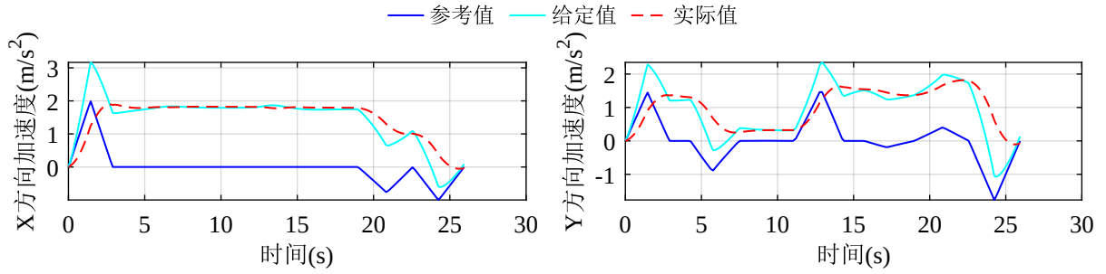
图 3-13 加速度曲线规划与跟踪结果
