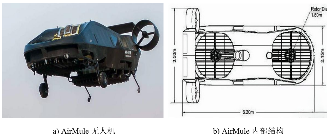
图 1-7 AirMule 无人机及内部结构
