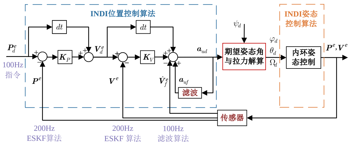
图 4-2 串级 INDI 抗扰控制系统框图
