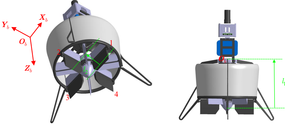
图 2-6 控制舵面及力臂示意图
