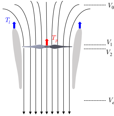
图 2-4 轴流状态的气动分析示意图
