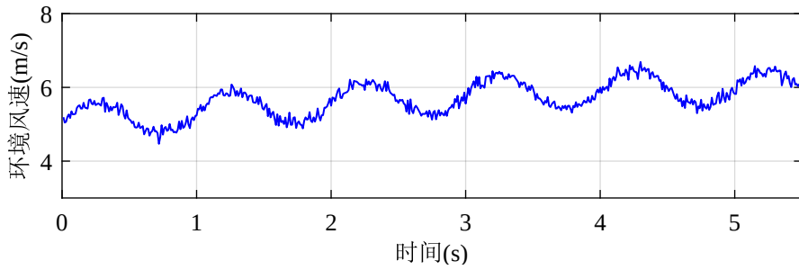
图 4-3 模拟环境风速扰动曲线
