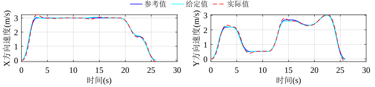
图 5-12 速度曲线规划与跟踪结果
