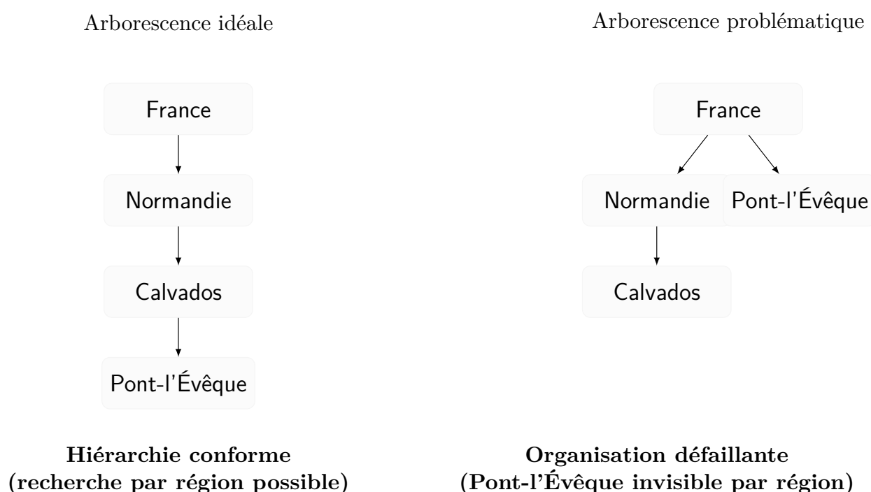
FIGURE 3.3 – Exemple de rattachement problématique dans le thésaurus : « Pont-l'Évêque » rattaché directement à « France », ce qui empêche sa remontée lors d'une recherche par région (« Normandie », « Calvados »).
