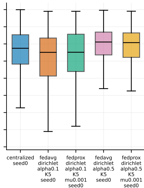
smoothgrad
