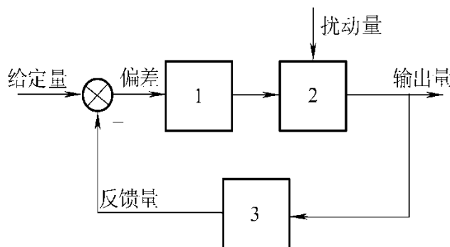
图 4-1 闭环系统示意图 [1]
