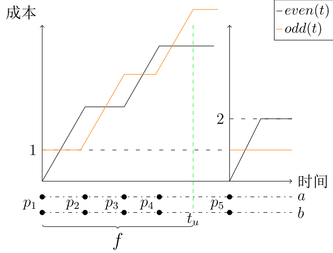
(a) 成本函数 odd(t) 和 even(t)
