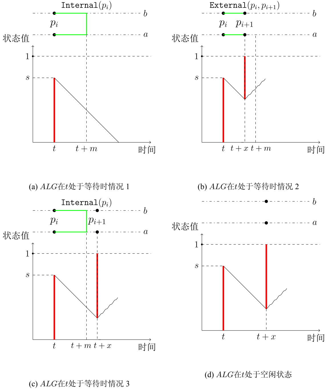
图 3.4 确定性算法 ALG 在 \tilde{R} 上的期望成本
