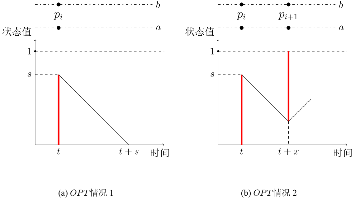
图 3.3 最优算法 OPT 在 \tilde{R} 上的期望成本
