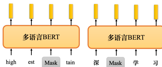
图 10.29 多语言 BERT
