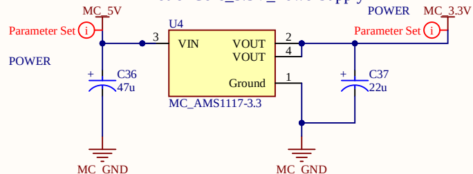
MotionCore_3.3V_PowerSupply
