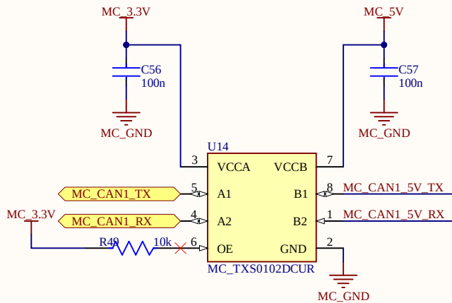
MotionCore_CAN_LogicShifter
